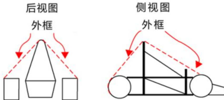
图 2.22 防滚架包络面
