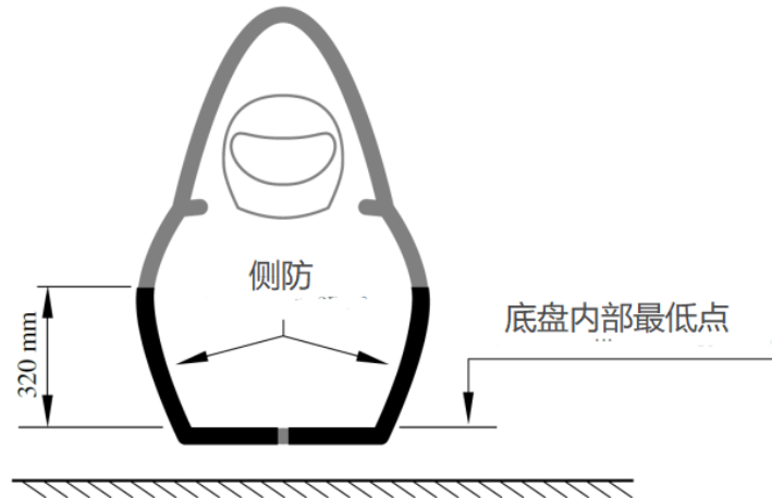
图 2.12 单体壳侧防区域
