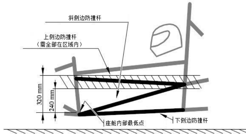
图 2.10 桁架式车架的侧边防撞结构
