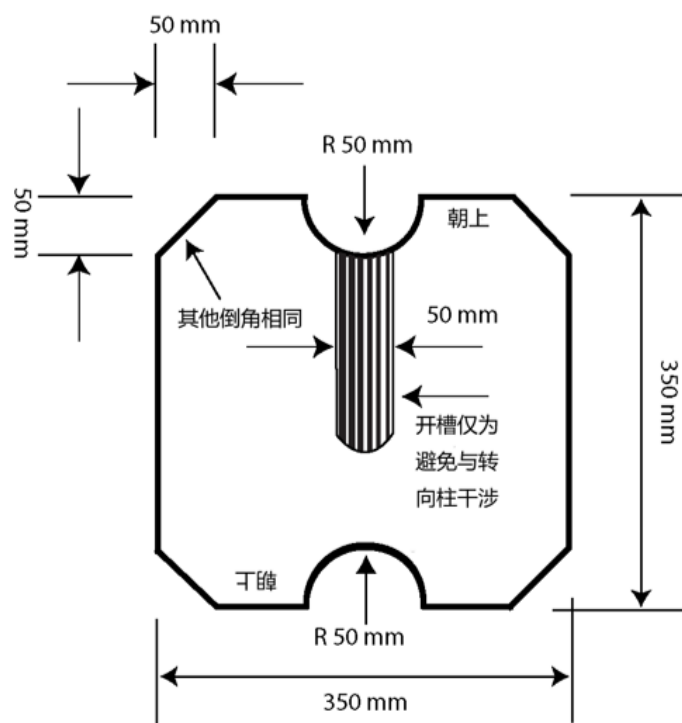
图 2.15 前舱检测板
