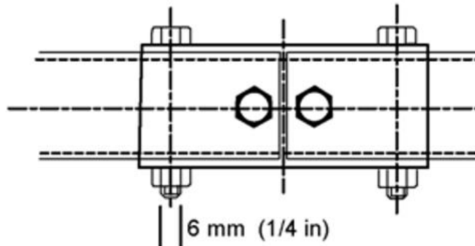
图 2.9 套管链接
