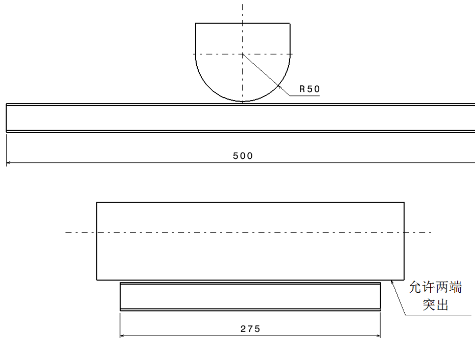
图 2.11 三点弯曲试验
