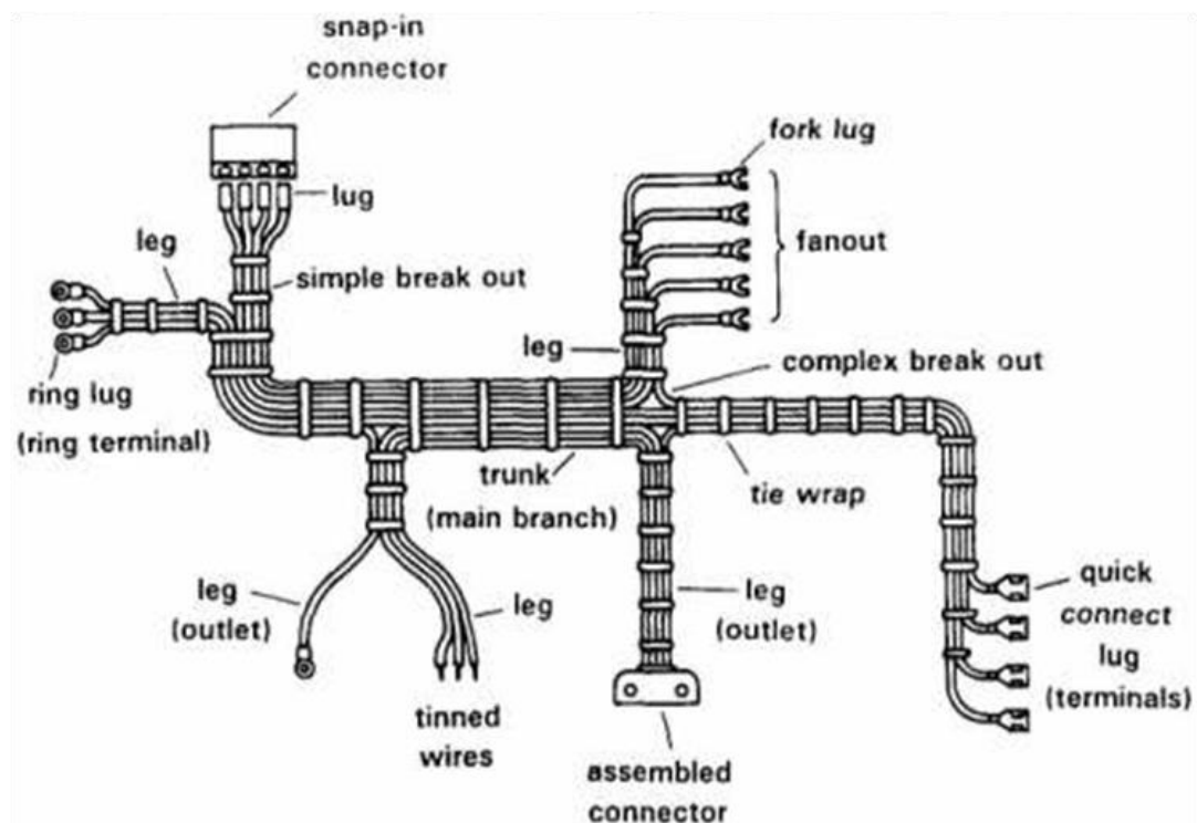
图 6.1 线束示意图
