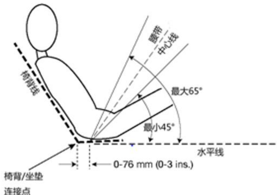
图 2.16 腰带的角度
