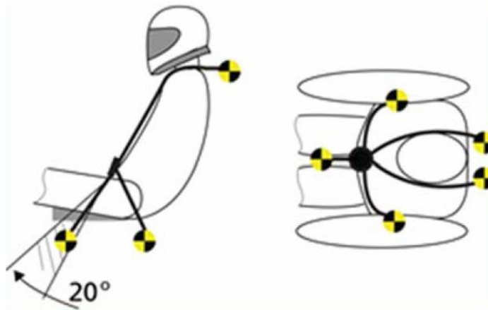
图 2.19 五点式安全带的反潜带安装图
