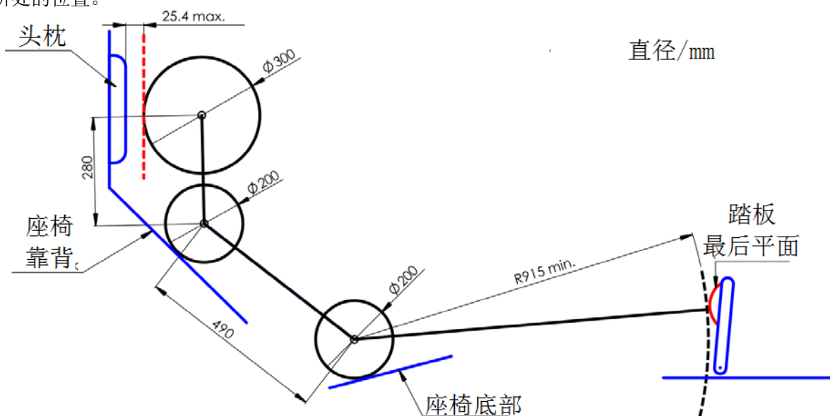
图 2.5 男性第 95 百分位模板位置
