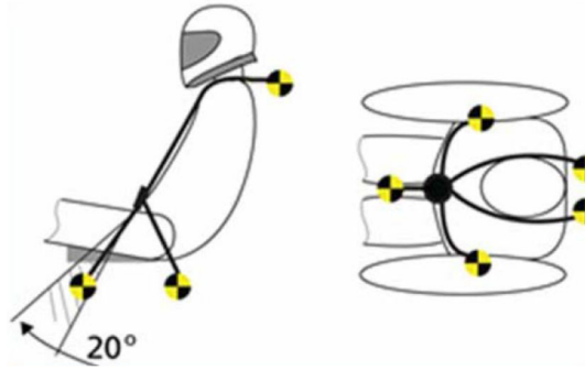
图 2.19: 五点式反潜带安装图
