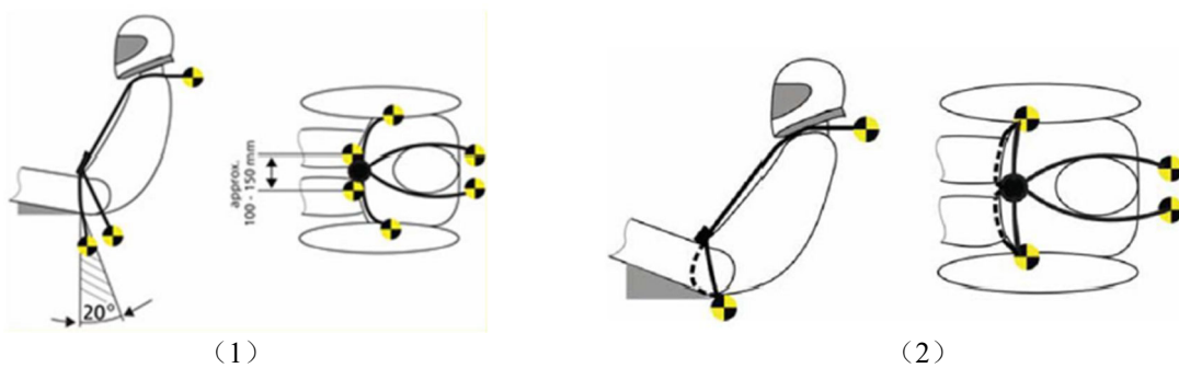
图 2.20: 六点式反潜带的两种安装图
