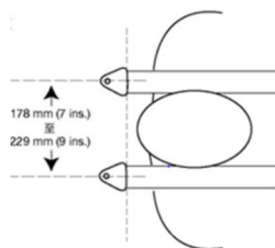
图 2.18: 肩带安装点
