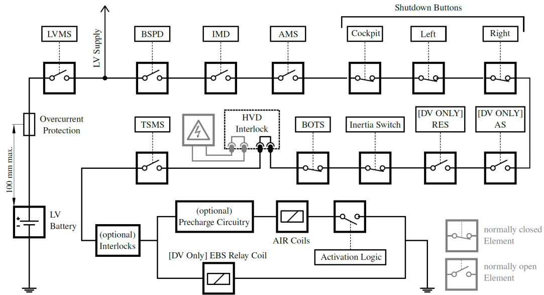
图 3.1: 安全回路的说明性原理示意图
