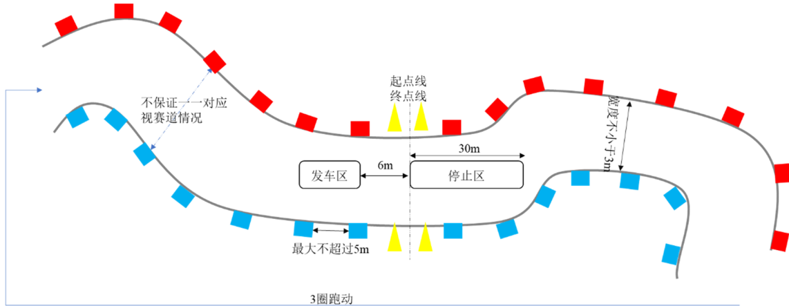
图 7.3: 高速循迹测试赛道示意图
