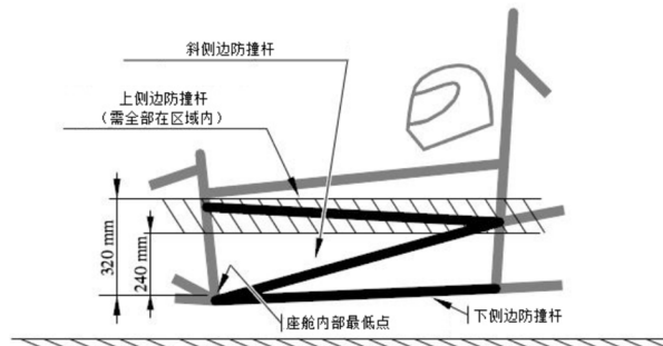
图 2.10: 侧防撞结构
