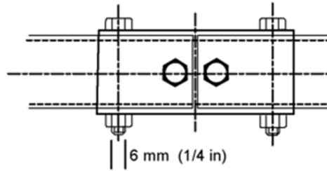
图 2.9: 套管连接
