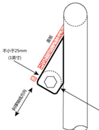
图 2.7: 双耳连接
