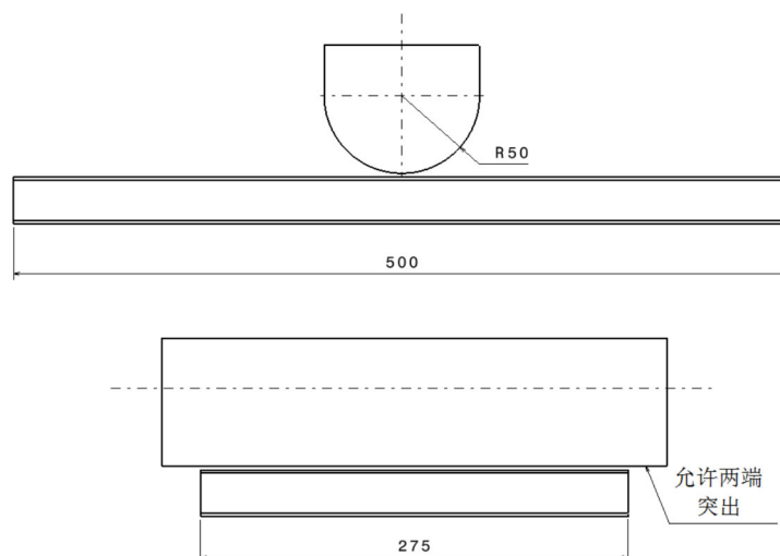
图 2.5: 三点弯曲试验
