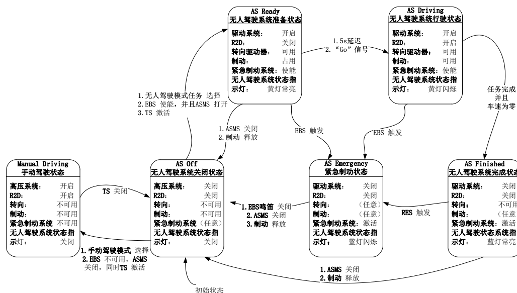
图 4.1: AS 状态机
