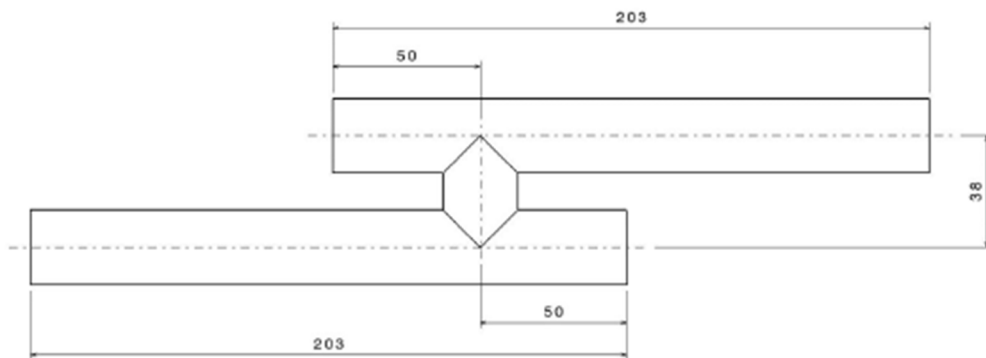
图 2.4: 测试样管示意图
