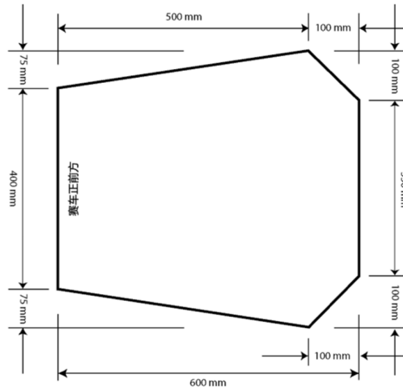
图 2.13: 驾驶舱开口检测板
