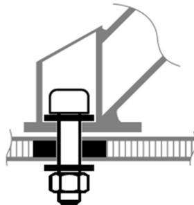
图 2.12：固定螺栓在管件中心线上
