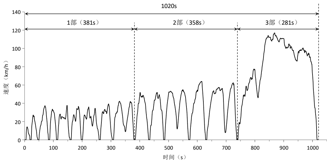
图2 激烈行驶工况曲线
