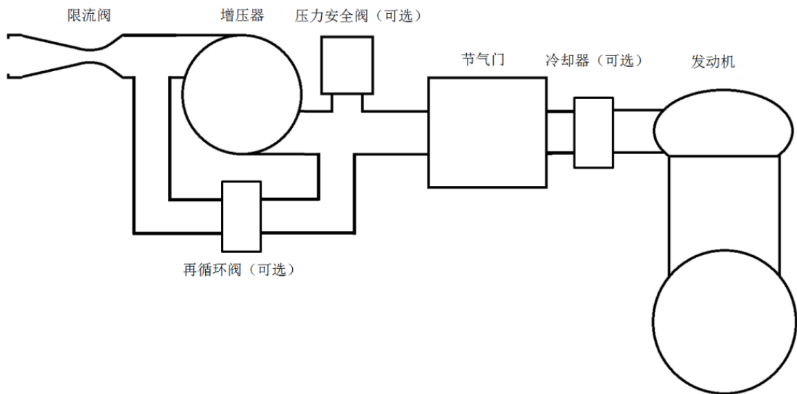
图 4.3 增压发动机进气顺序
