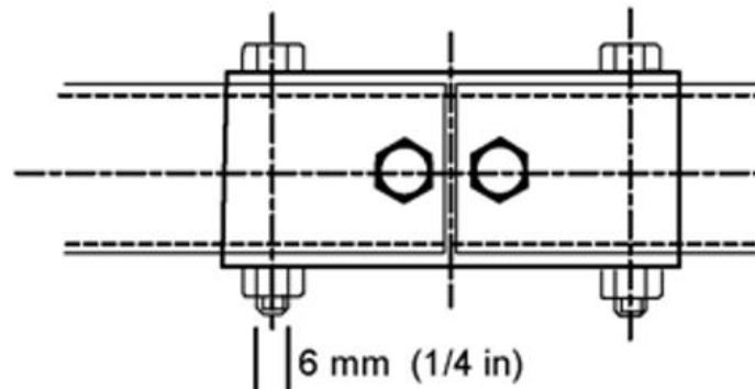
图 2.9 套管链接
