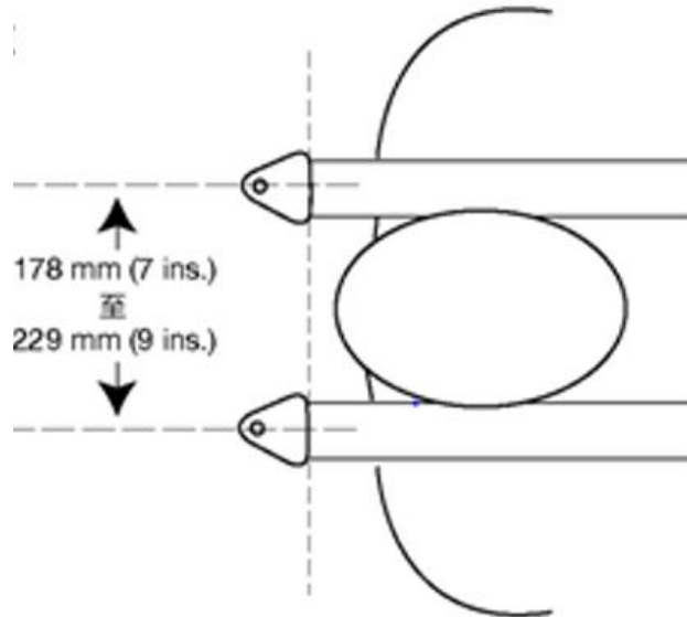
图 2.17 肩带安装点
