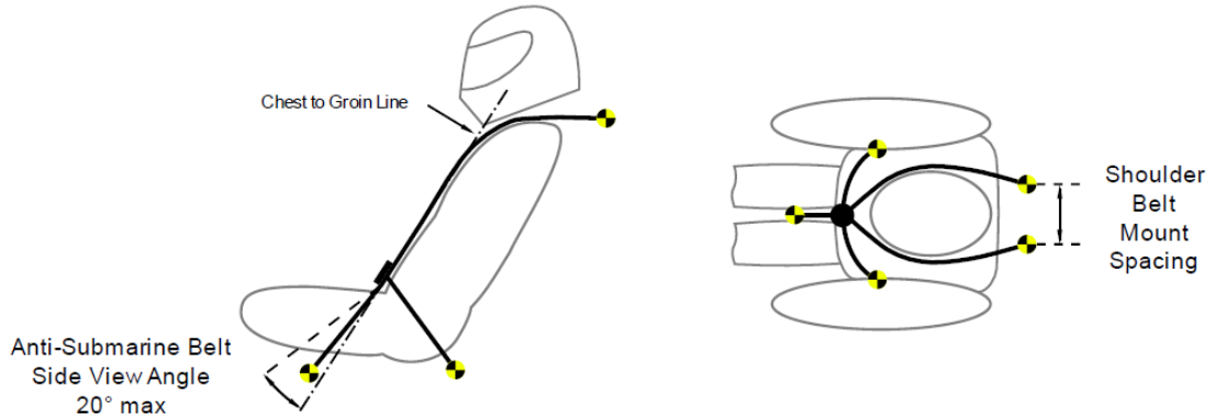
图 2.19 五点式安全带的反潜带安装图
