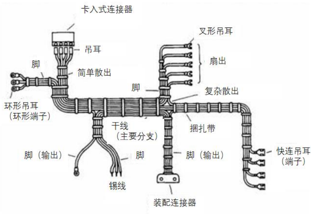
图 6.1 线束示意图
