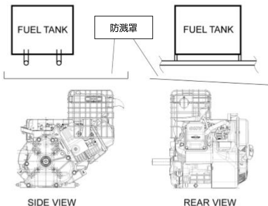
图B-44：燃料系统，防溅罩安装示例
