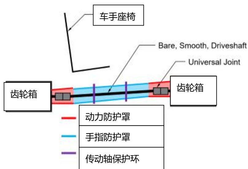
图B-52:传动轴保护
