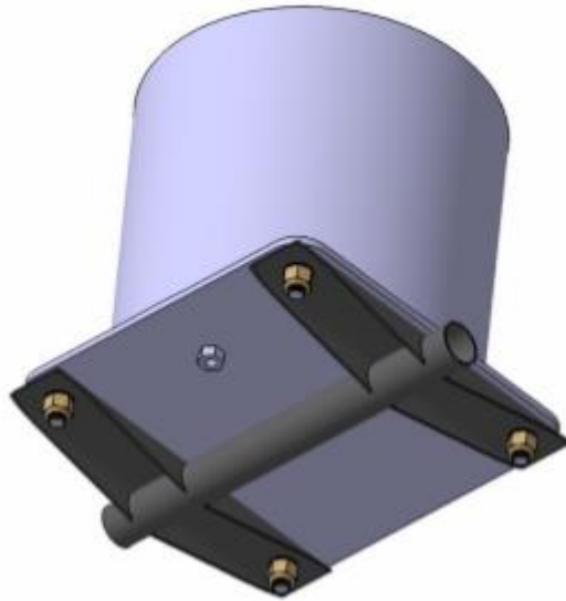
图B-41：安装在“C”支架上的油箱。(可接受的安装设计)
