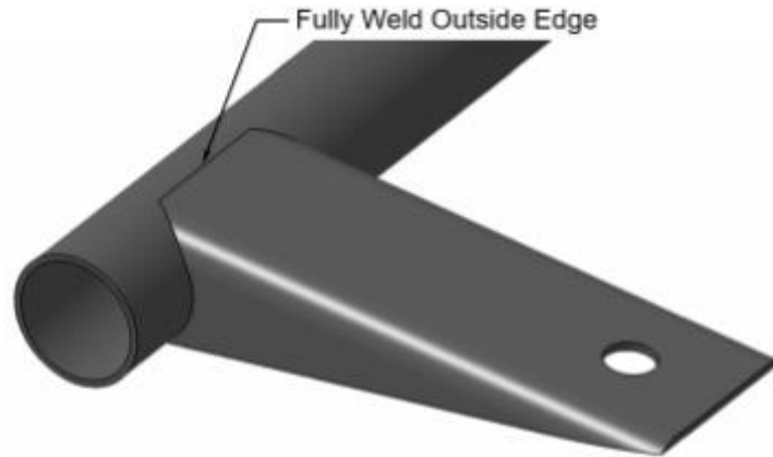
图B-43：最小焊接长度
