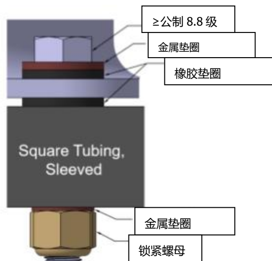
图B-39：油箱紧固件堆叠
