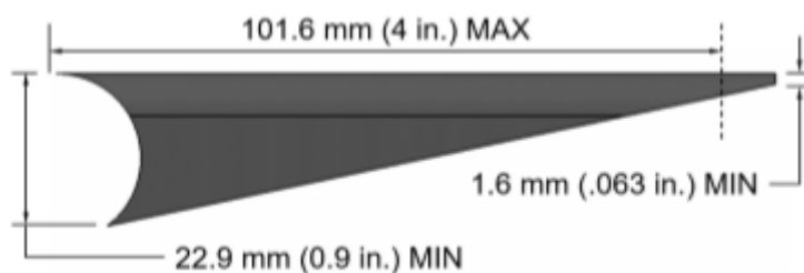
图B-42：允许锥度
