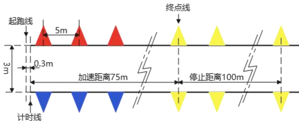
图 7.3: 直线赛道示意图
