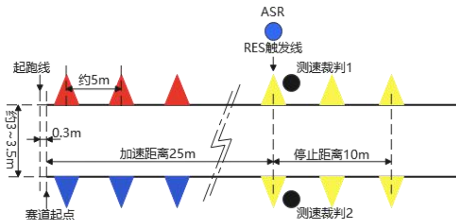
图 5.1 紧急制动测试赛道示意图
