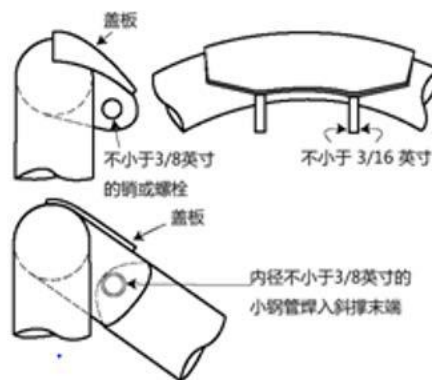
图 2.8: 双耳连接
