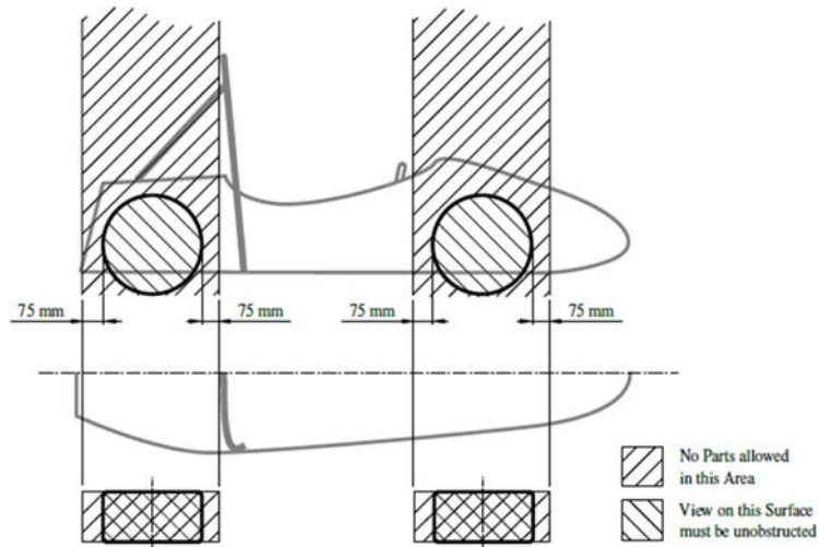
图 2.3: 车轮周围排除区
