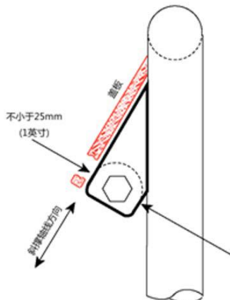
图 2.7: 双耳连接
