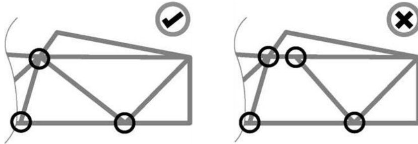
图 2.1: 车架单元的点对点三角结构（左侧正确、右侧错误）
