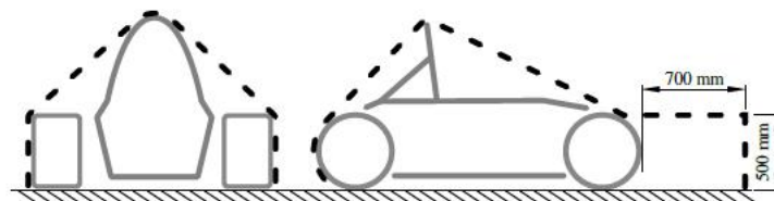
图 4.4 传感器安装位置
