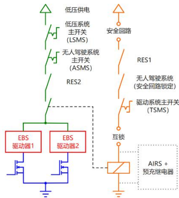
图 4.3 EBS 电气原理图
