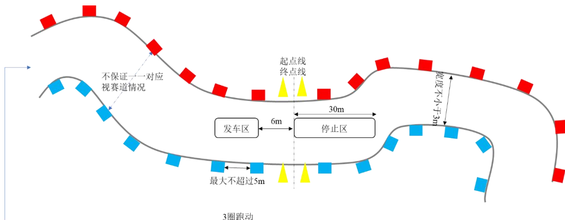
图 7.4: 高速循迹测试赛道示意图
