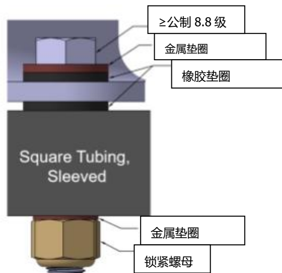
图B-2：油箱紧固件堆叠
