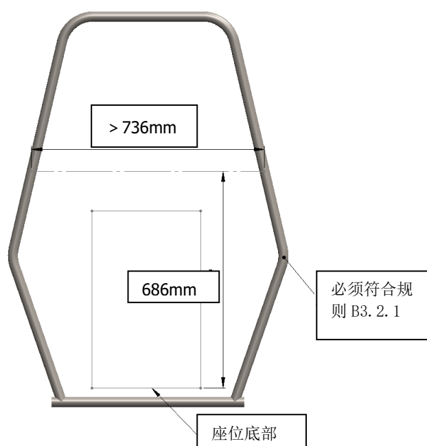
图B-15：防滚架 RRH
