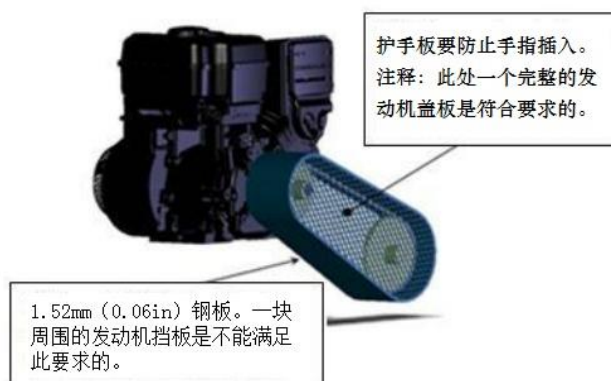
图B-51: CVT上的动力系统保护范围示例
