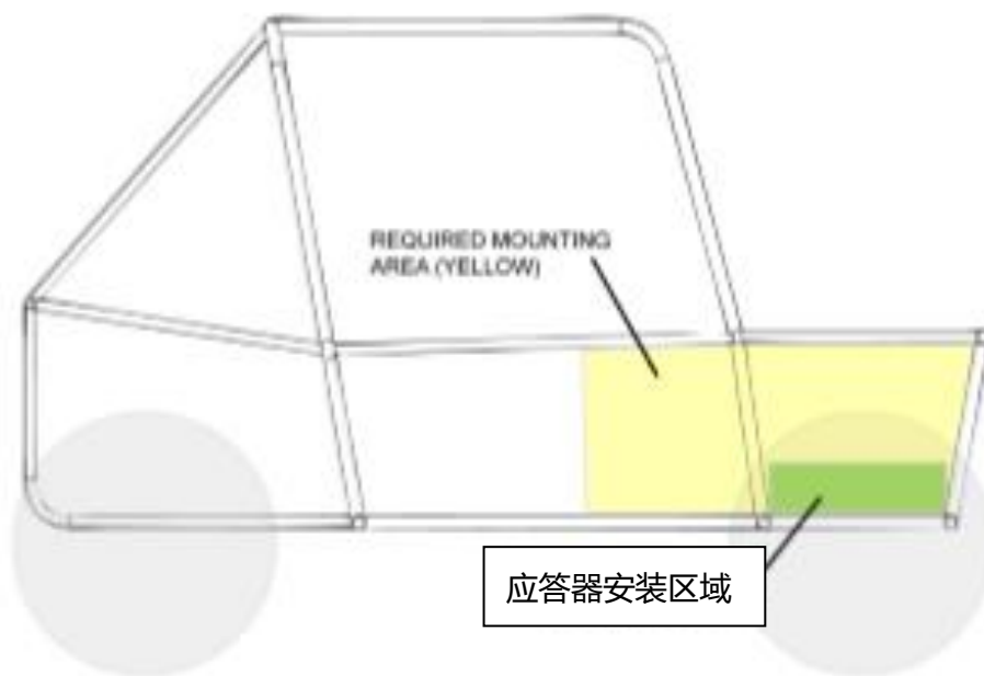
图B-65:应答器，安装位置
