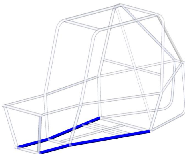
图B-21：防滚架后支撑框架模式 LFS
