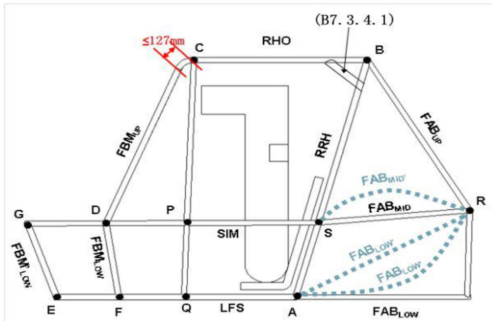
图B-26：防滚架FAB
