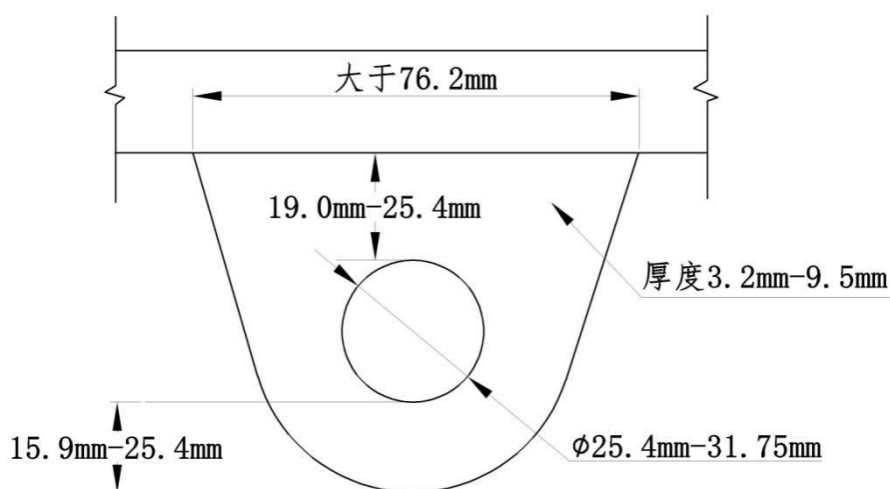
图B-58：后悬挂点尺寸图
