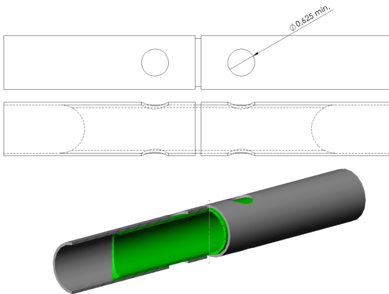
图B-27：滚筒式保持架，对接套筒
