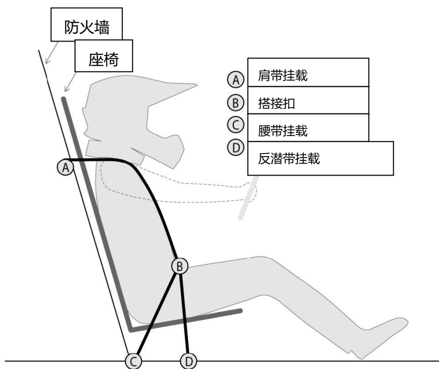
图B-33：安全带约束示意图
