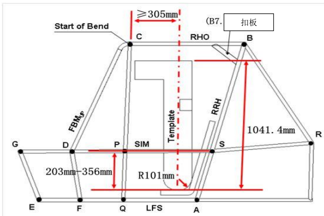
图B-18: 防滚架 模板安装图
