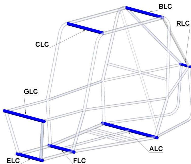
图B-14: 防滚架横向横梁
