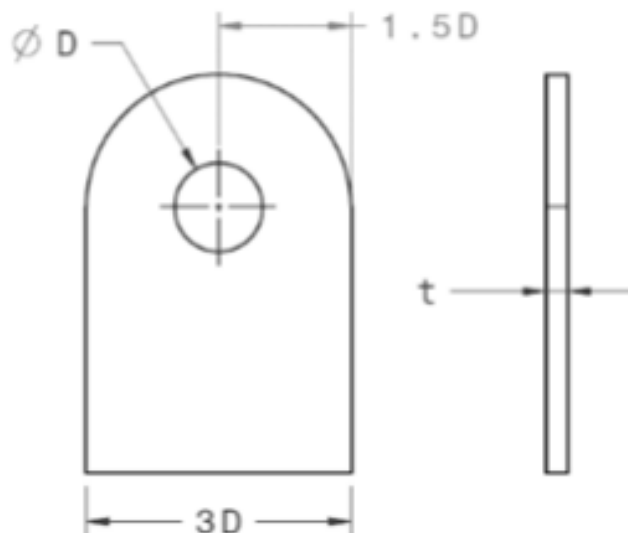
图B-60：吊耳制作比例图
