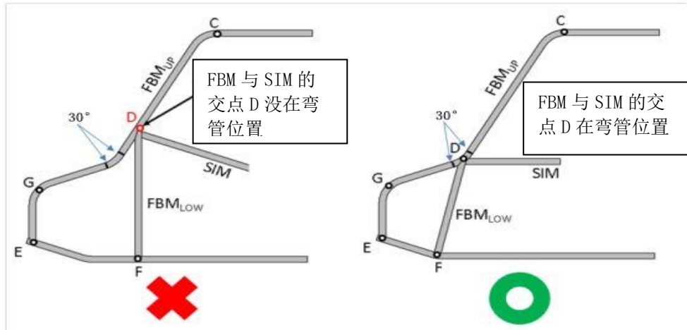
图B-9：防滚架弯管交点位置
