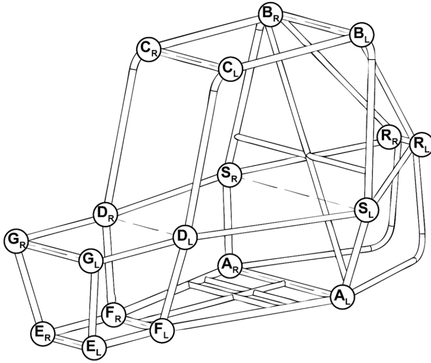
图B-12: 防滚架命名点 (后支撑框架模式)
