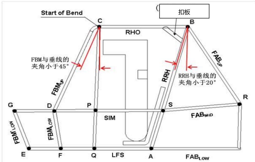
图B-24：防滚架FBM
