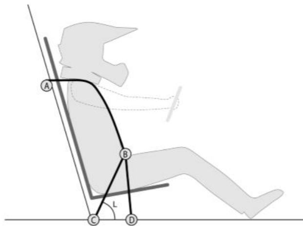
图B-39: 车手安全腰带角度
