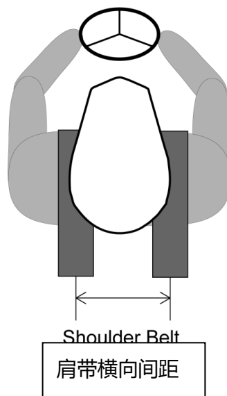
图B-36：驾驶员背带、肩带横向位置
