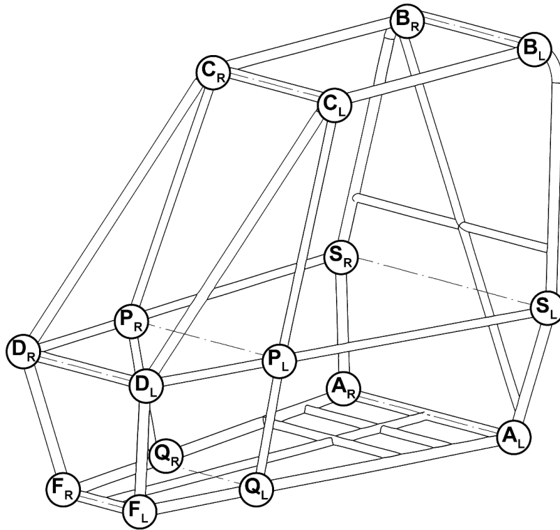
图B-13: 防滚架命名点 (前支撑框架模式)
