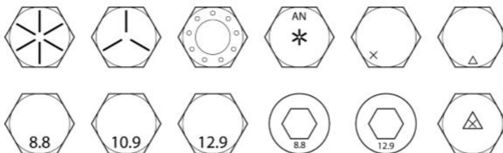
图B-59 紧固件，可接受的标记
