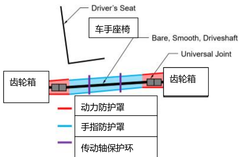
图B-54: 传动轴保护
