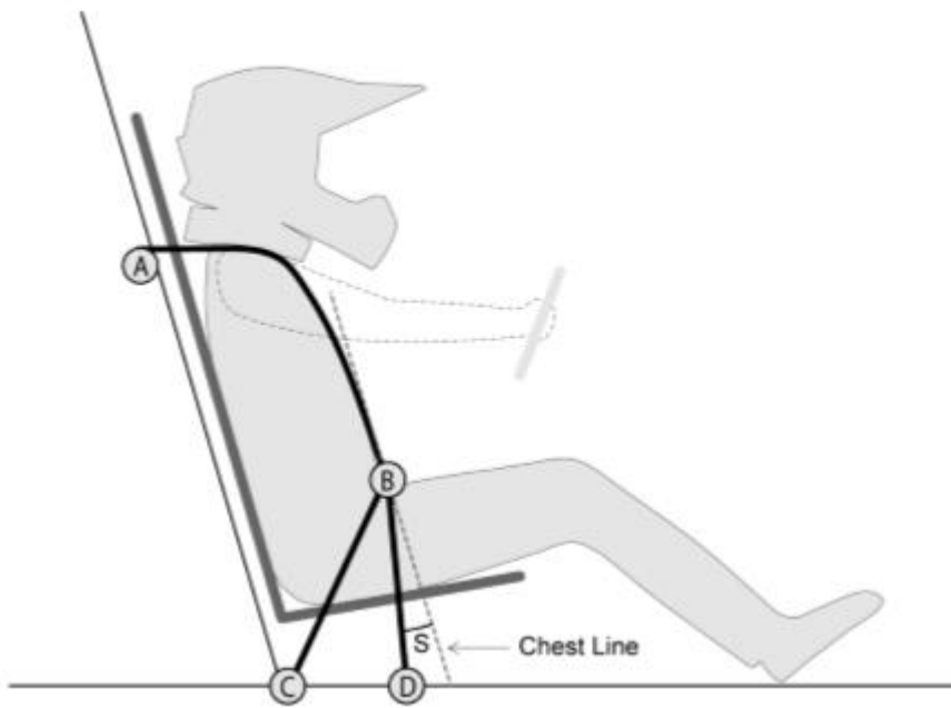
图B-41：车手安全带，反潜带角度
