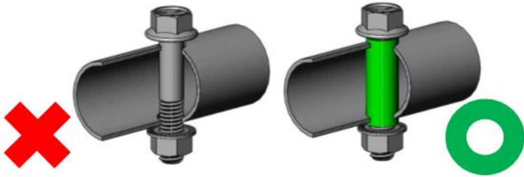
图 B-32: 防滚架套管连接
