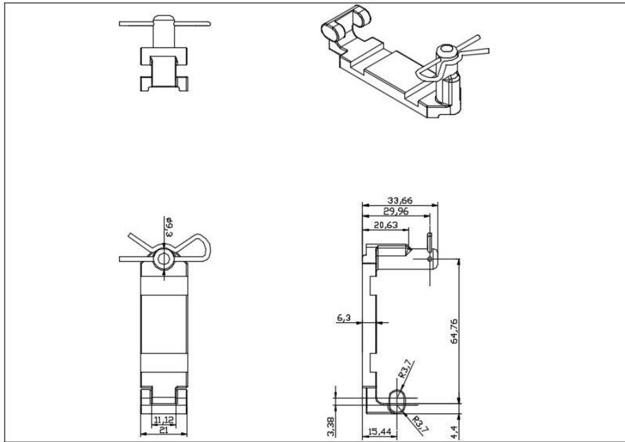
图B-66：应答器固定支架
