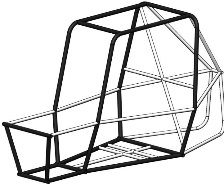
图B-11：防滚架主要结构件(黑色填充)，后支撑框架模式
