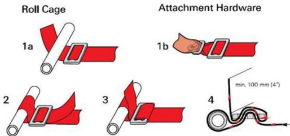
图B-38：安全带织带正确缠绕示意图
