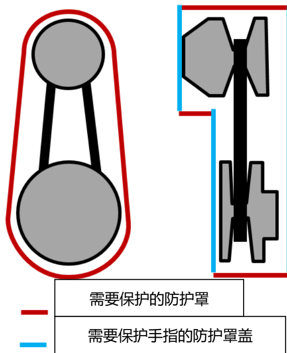
图B-51: CVT上的动力系统保护范围示例
