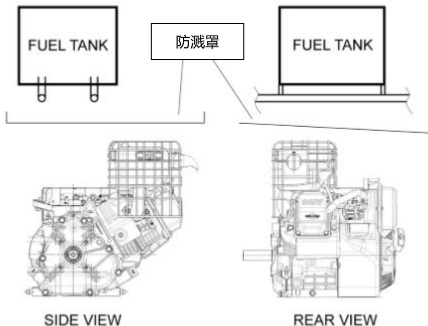
图B-7：燃料系统，防溅罩安装示例
