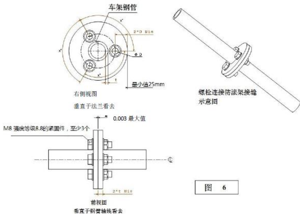
图B-31:螺栓连接防滚架
