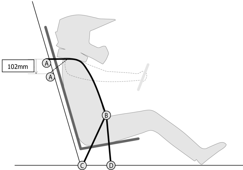
图B-35：安全带肩带垂直位置
