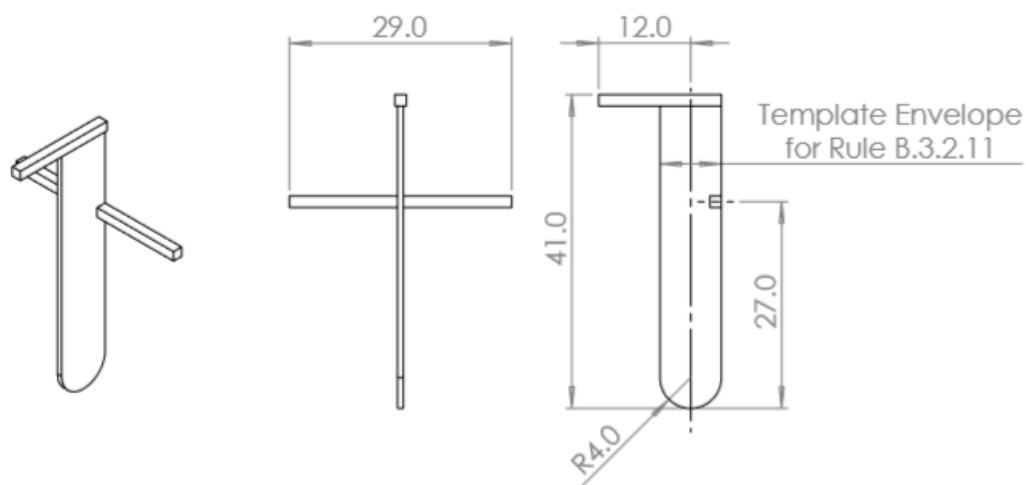
图B-19: 防滚架模板图
