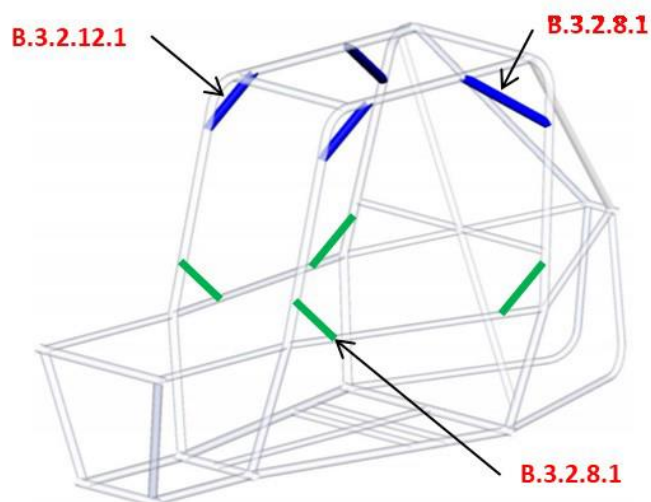
图B-20：防滚架支撑件
