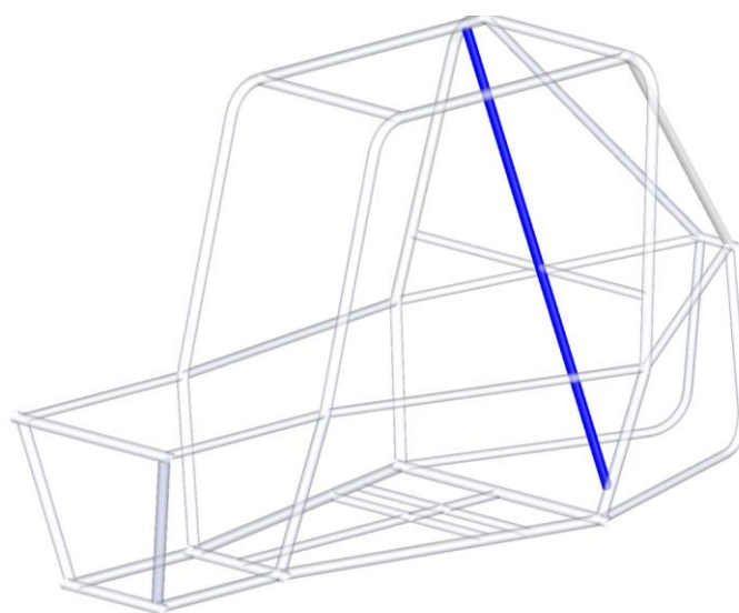
图B-16：防滚架 LDB
