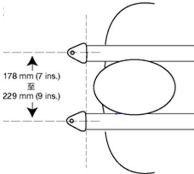
图 2.17 肩带安装点
