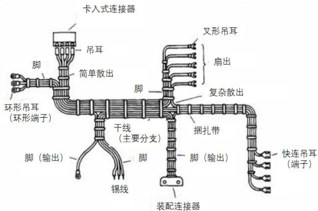
图 6.1 线束示意图
