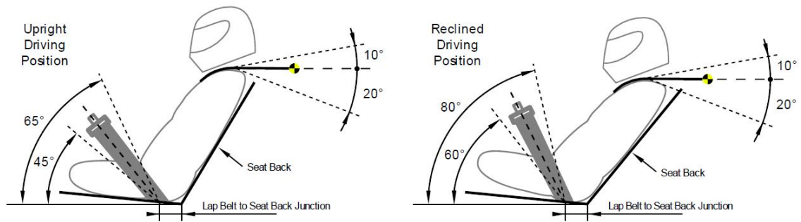
图 2.18 肩带安装角
