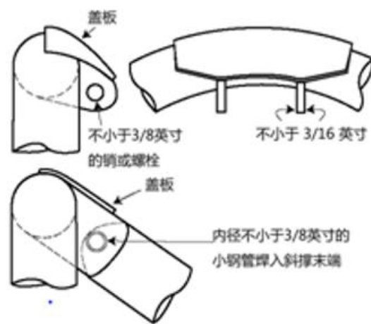
图 2.8 双耳连接
