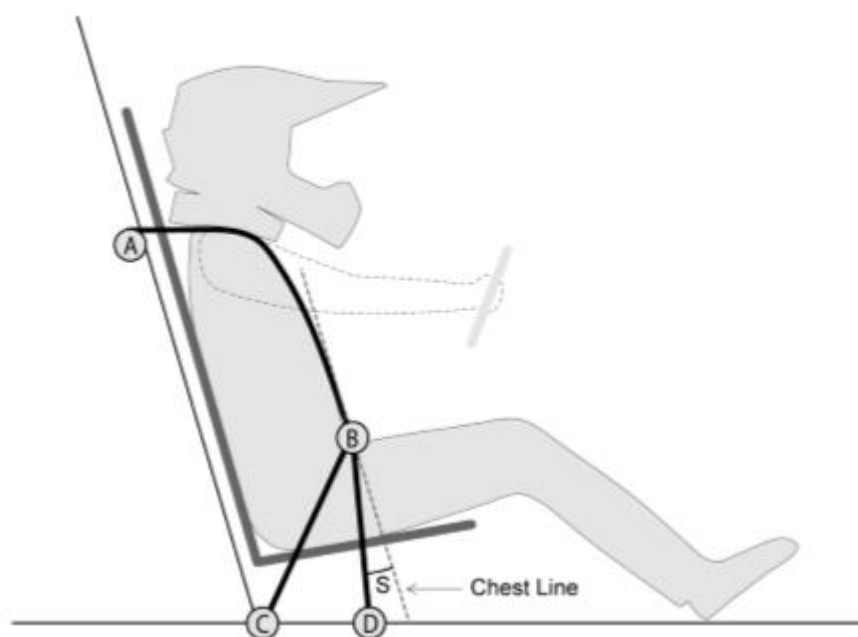
图B-48 车手安全带，反潜带角度
