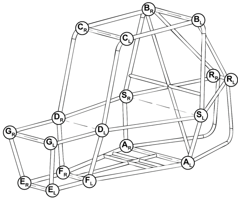
图B-18 防滚架示例、定义点、带“鼻”、后支撑
