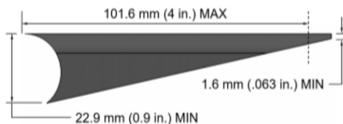
图B-7 允许锥度
