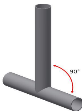
图B-34 防滚架焊接试样1
