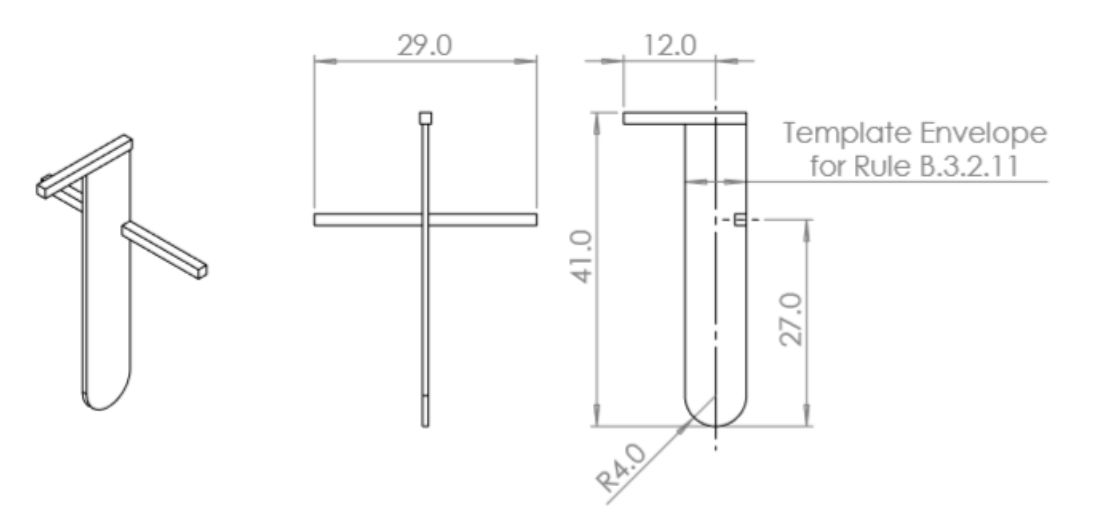
图B-25 防滚架模板图
