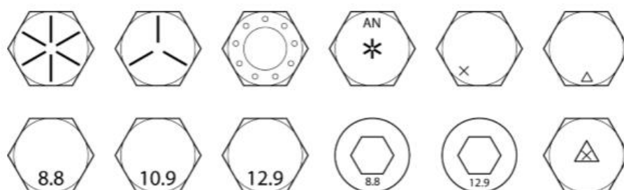
图B-68 紧固件，可接受的标记
