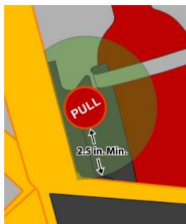
图B-58 灭火器，拉手周围间隙示意图(绿色)
