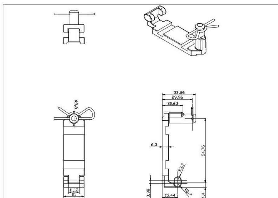
图B-75 应答器固定支架
