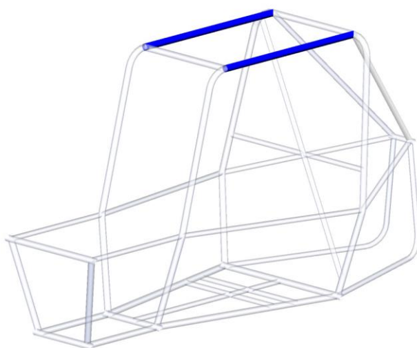
图B-23 防滚架 RH0
