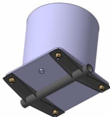
图B-6 安装在“C”支架上的油箱。（可接受的安装设计）
