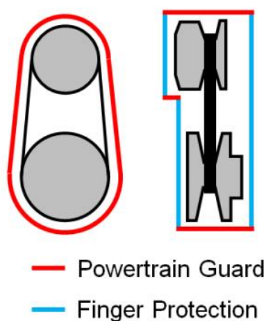
图 B-63 CVT 防护罩
