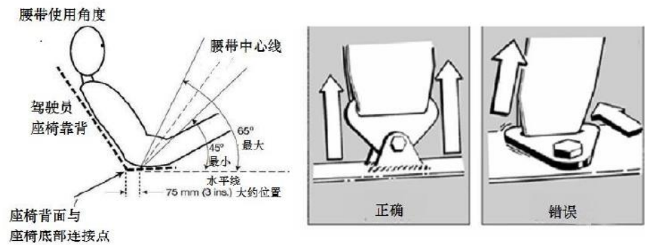
图B-47 车手安全带 搭扣方向
