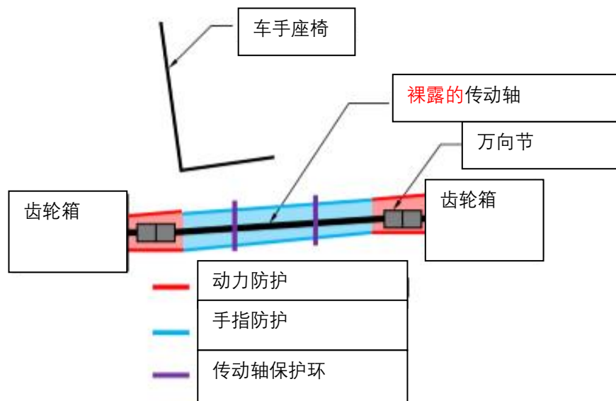
图B-60 传动轴动力保护示例
