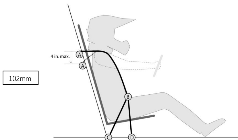
图B-42 安全带肩带垂直位置
