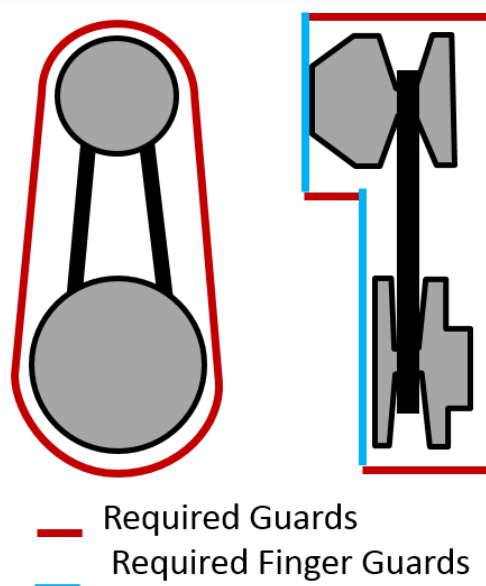
图B-59 CVT动力保护示例
