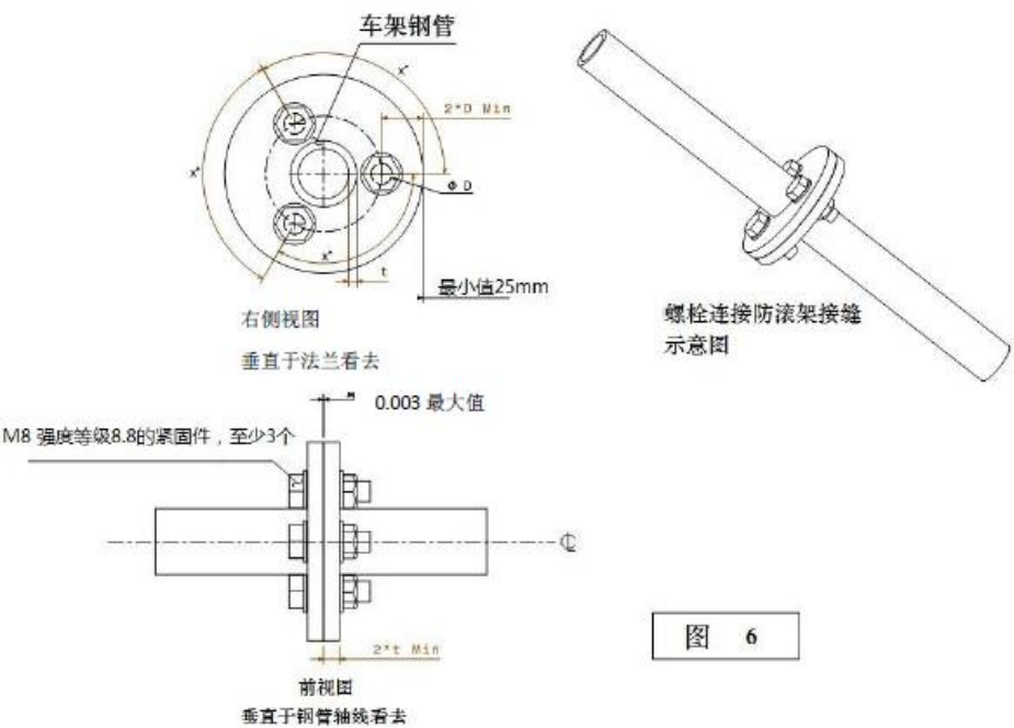
图B-37 螺栓连接防滚架
