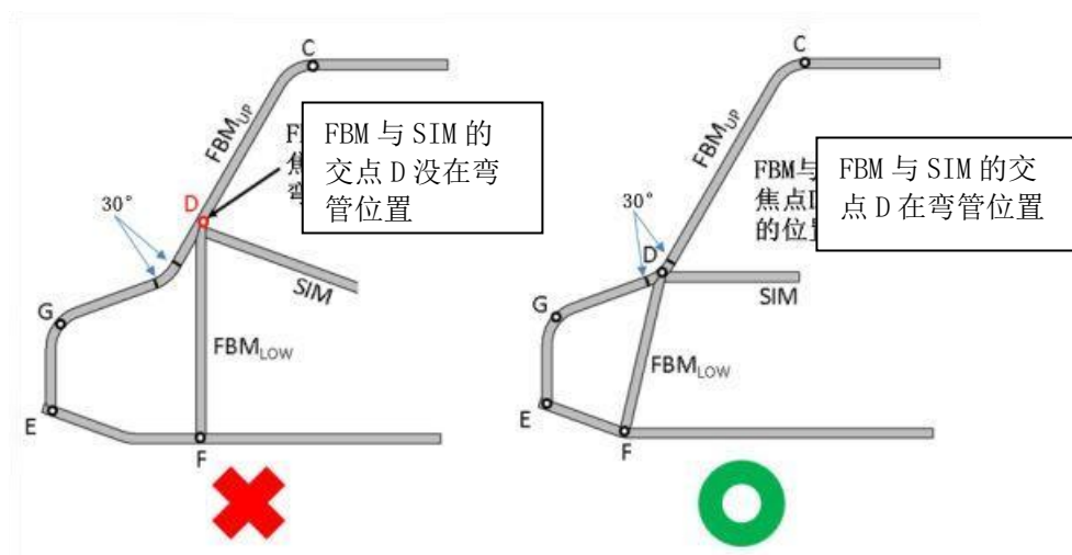
图B-15 防滚架弯管交点位置
