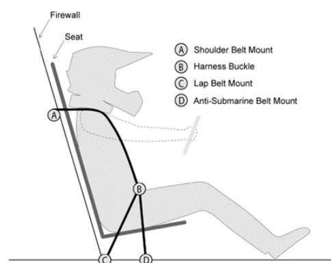
图B-39 安全带约束示意图
