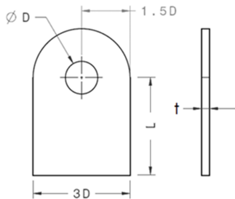
图B-69 吊耳图
