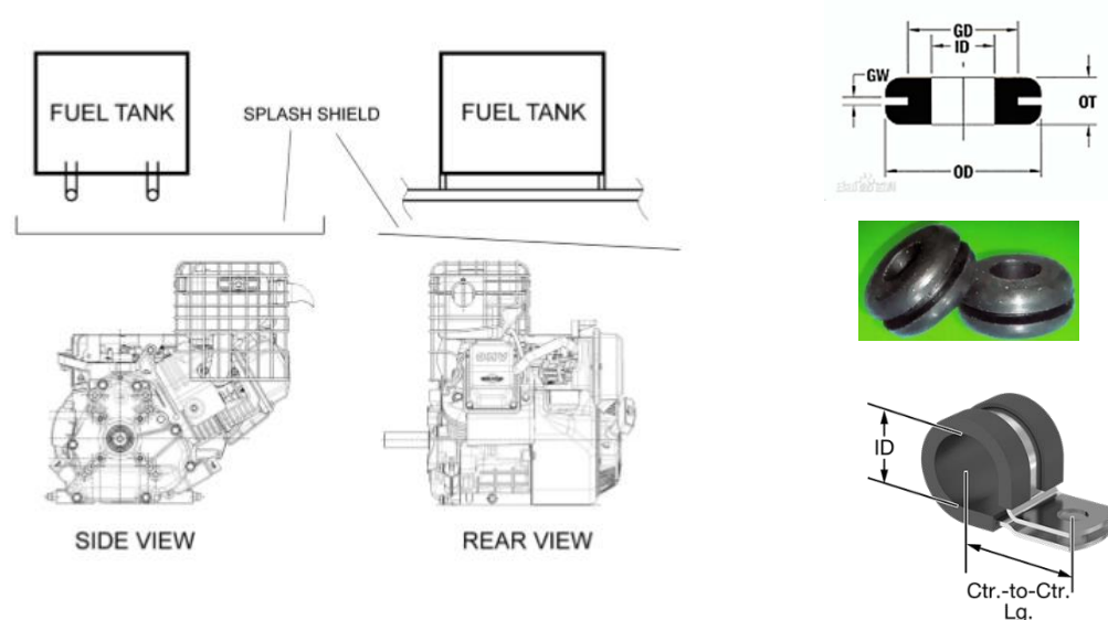
图B-9 防溅罩安装示例
