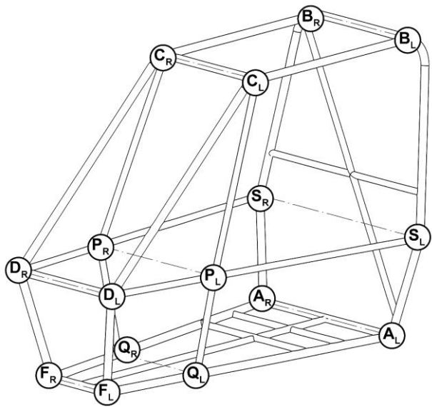
图B-19 防滚架示例、定义点、前支撑
