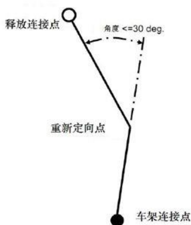
图B-49 反潜带重定向
