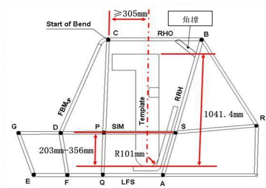
图B-24 防滚架 模板安装图
