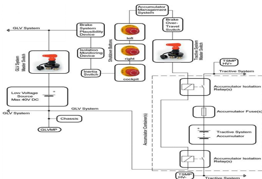
图B-12 安全回路原理图
