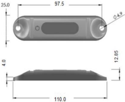
图B-78 RFID标签尺寸
