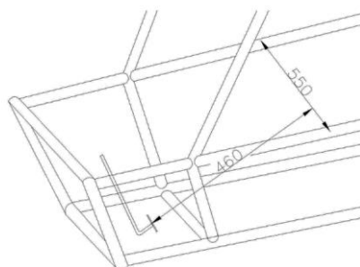
图B-36：测量横向空间距离示意图
