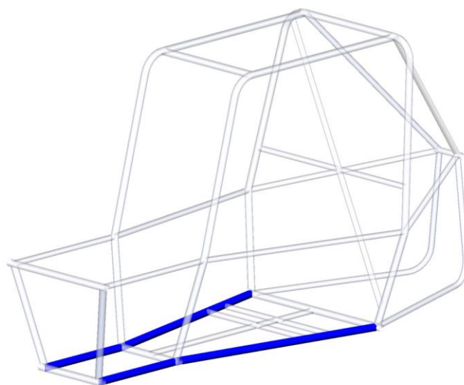
图B-27 防滚架后支撑车架模式 LFS
