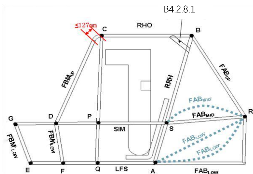
图B-32防滚架FAB
