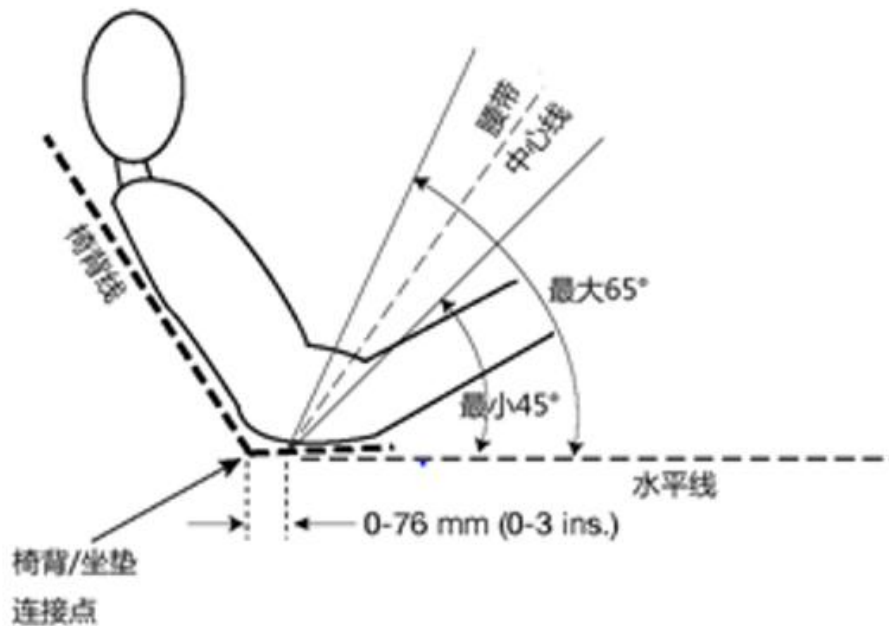
图 2.16 腰带的角度
