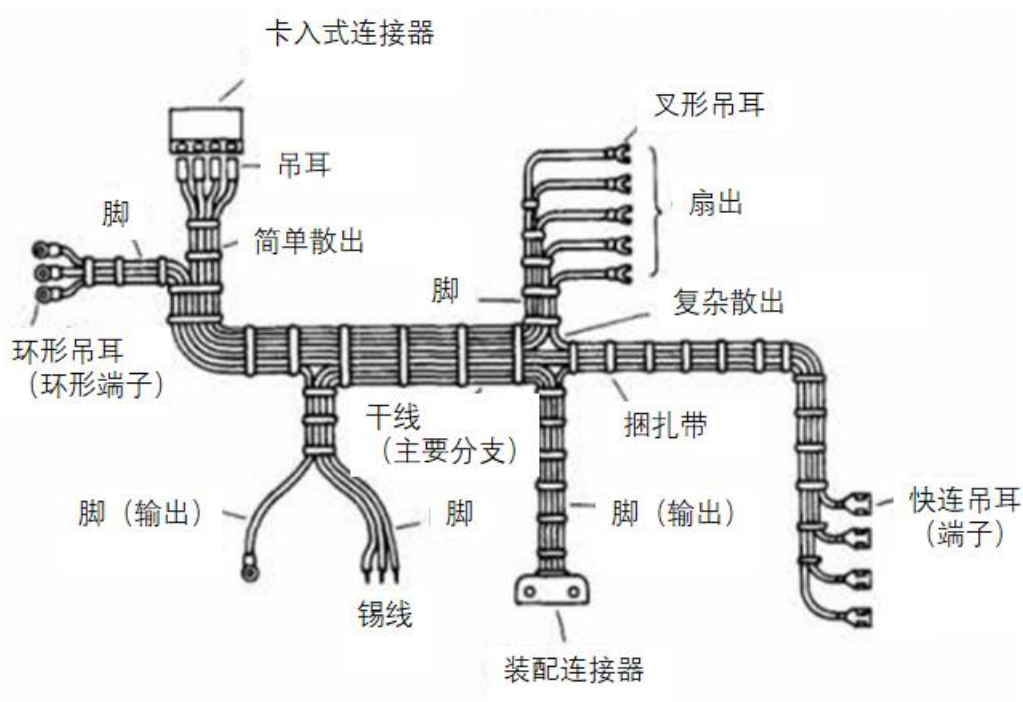
图 7.1 线束示意图
