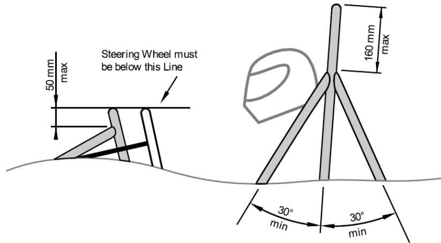
图 2.9 防滚架位置要求
