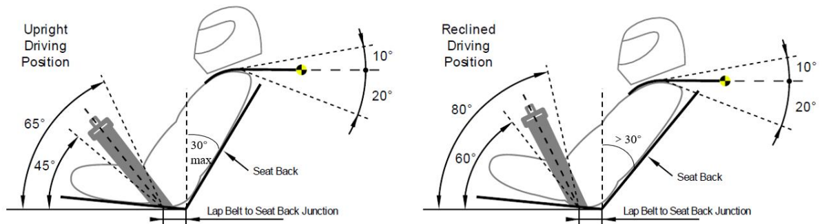
图 2.18 肩带安装角
