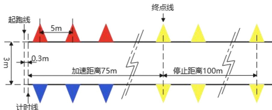
图 8.2 无人直线赛道示意图
