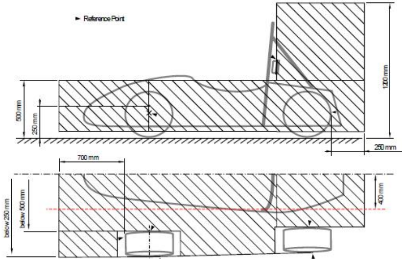
图2.26 空气动力学区域
