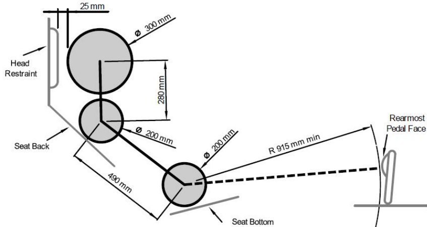
图 2.8 男性第 95 百分位模板位置
