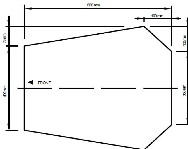
图 2.14 座舱检测板
