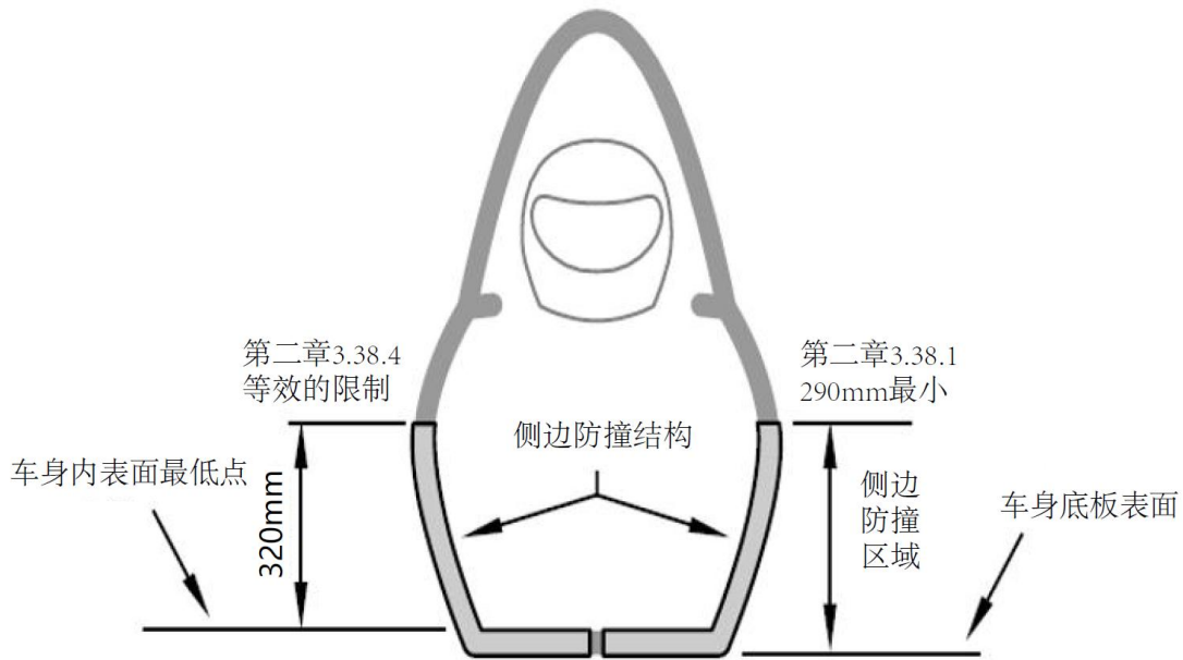
图 2.12 单体壳侧边防撞区域
