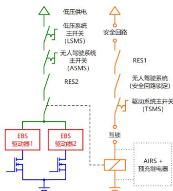
图 4.3 EBS 电气原理图
