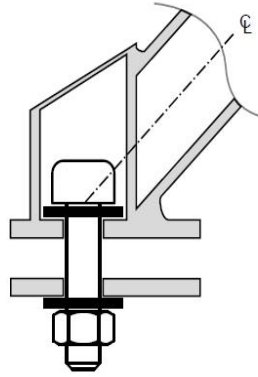
图 2.13 固定螺栓在管件中心线上
