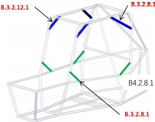
图B-26 防滚架角支撑
