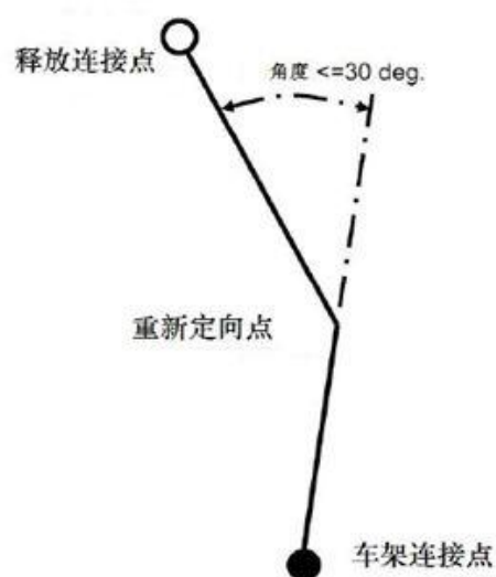
图B-49 反潜带重定向
