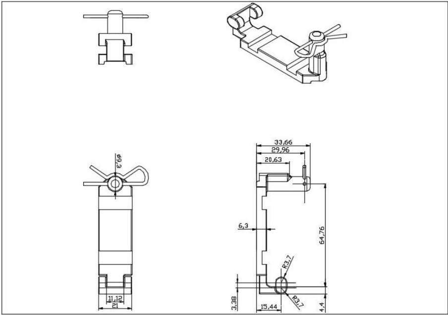
图B-76 应答器固定支架
