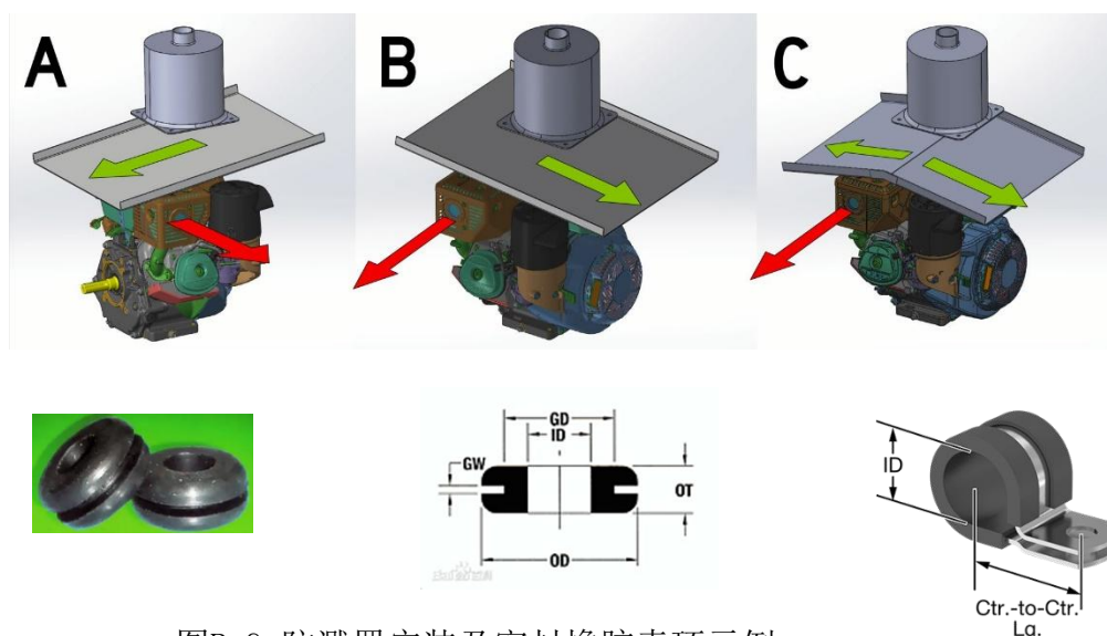
图B-9 防溅罩安装及密封橡胶索环示例
