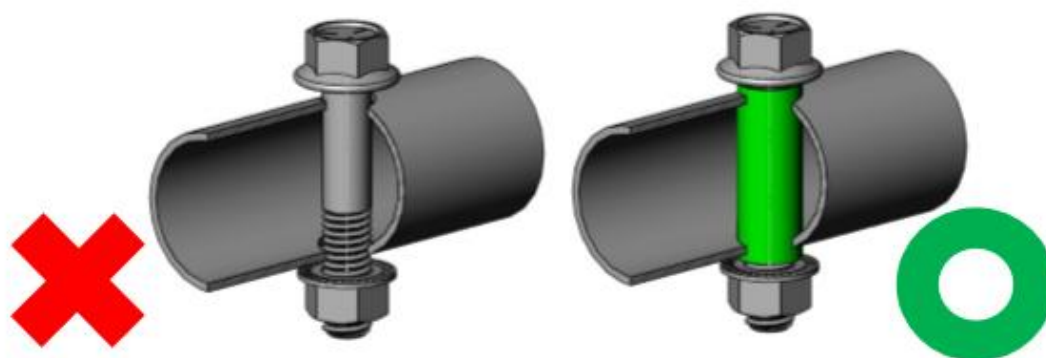
图 B-38 防滚架套管连接
