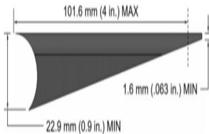
图B-7 允许锥度
