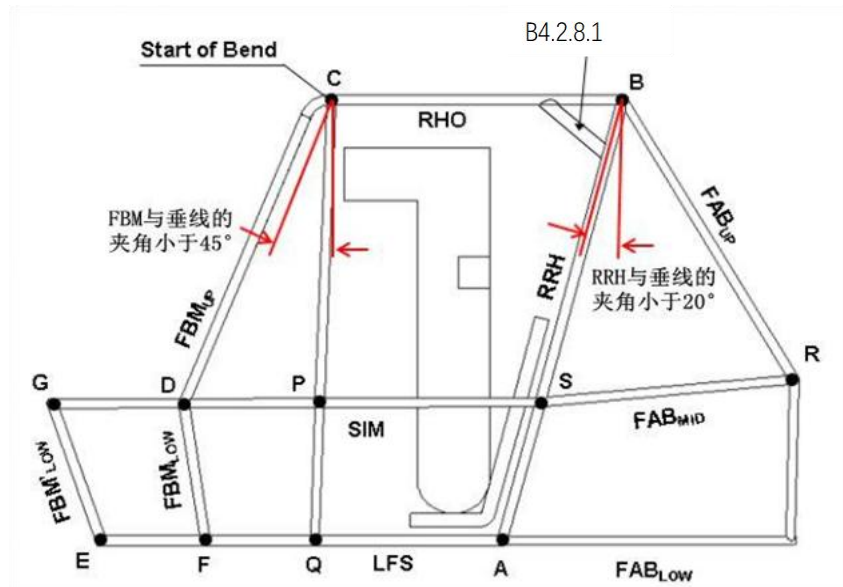
图B-30 防滚架FBM
