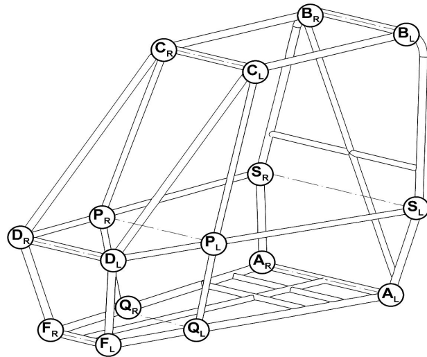
图B-19 防滚架示例、定义点、前支撑
