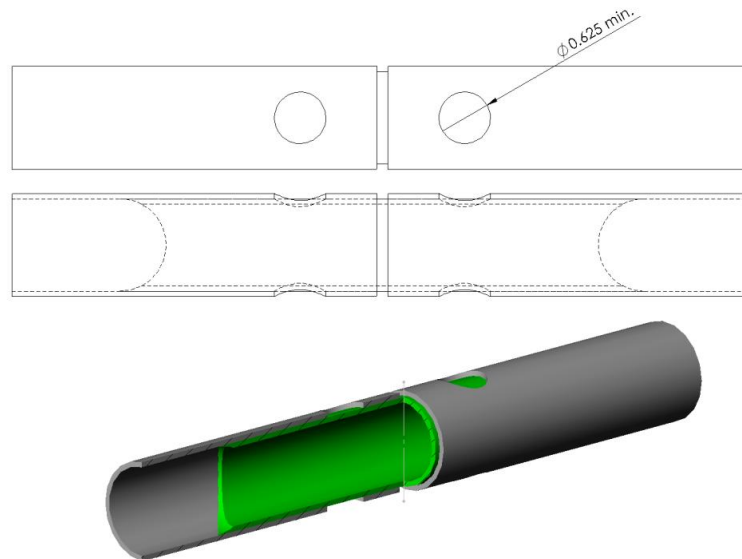
图B-33 防滚架，对接套筒
