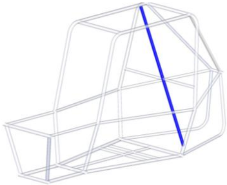
图B-22 防滚架侧撑构件LDB
