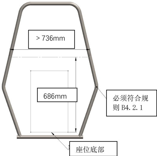
图B-21 防滚架 RRH
