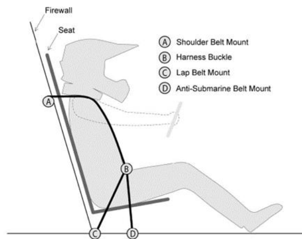
图B-39 安全带约束示意图
