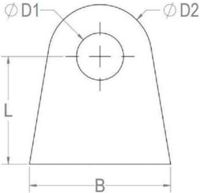
图B-70 吊耳几何形状
