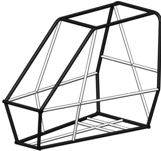
图B-16 防滚架主要构件(黑色填充)，前支撑车架模式
