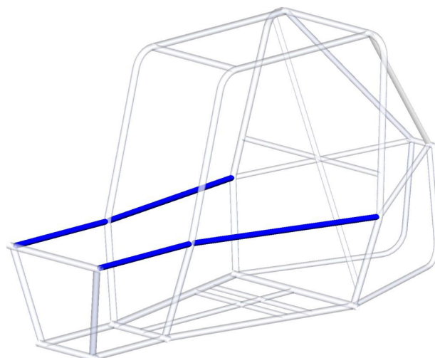
图B-28 防滚架后支撑车架模式 SIM
