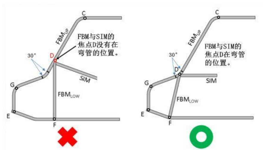
图B-15 防滚架弯管交点位置
