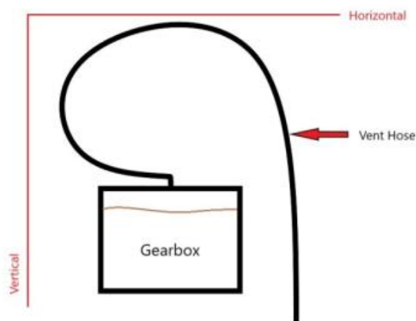
图B-62 变速箱通风系统（水平=从左到右）
