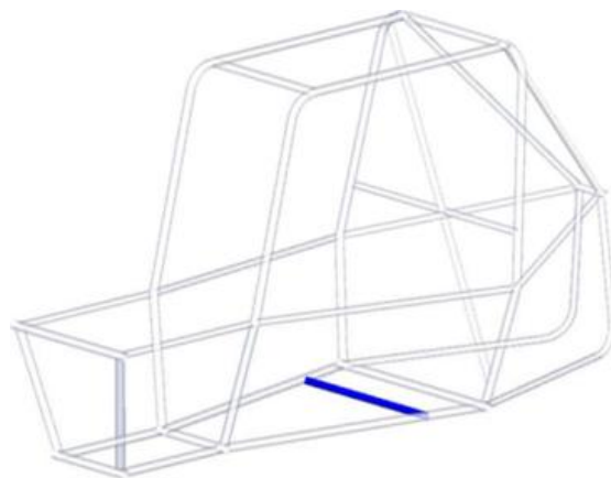
图B-29 防滚架USM范例
