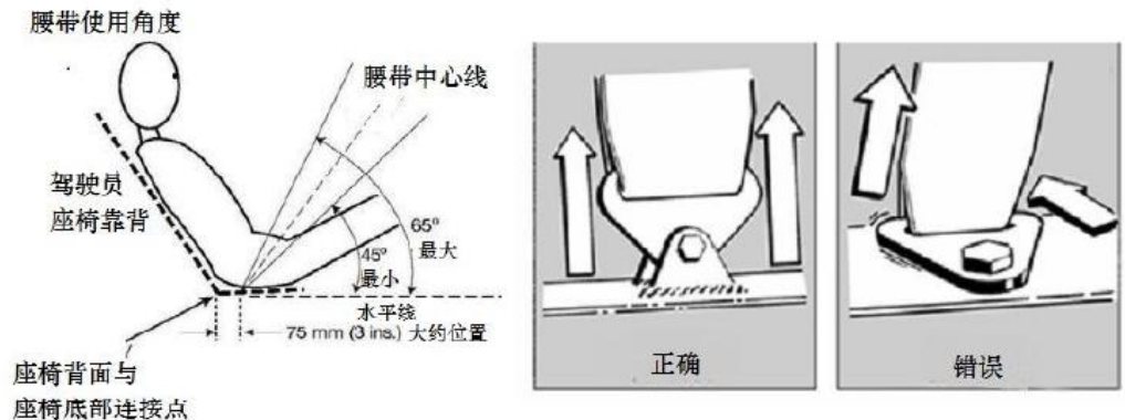
图B-47 车手安全带 搭扣方向
