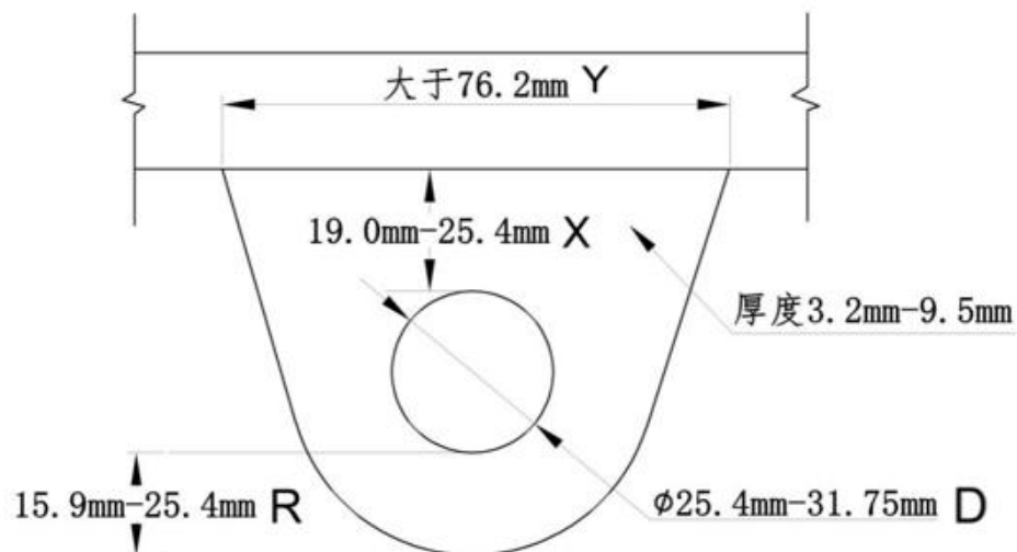
图B-67 后拖拽点尺寸图
