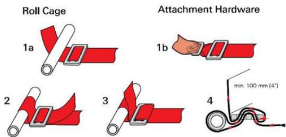
图B-45 安全带织带正确缠绕示意图
