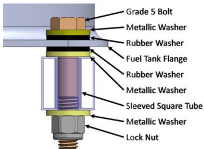
图B-4 油箱紧固件安装示意图
