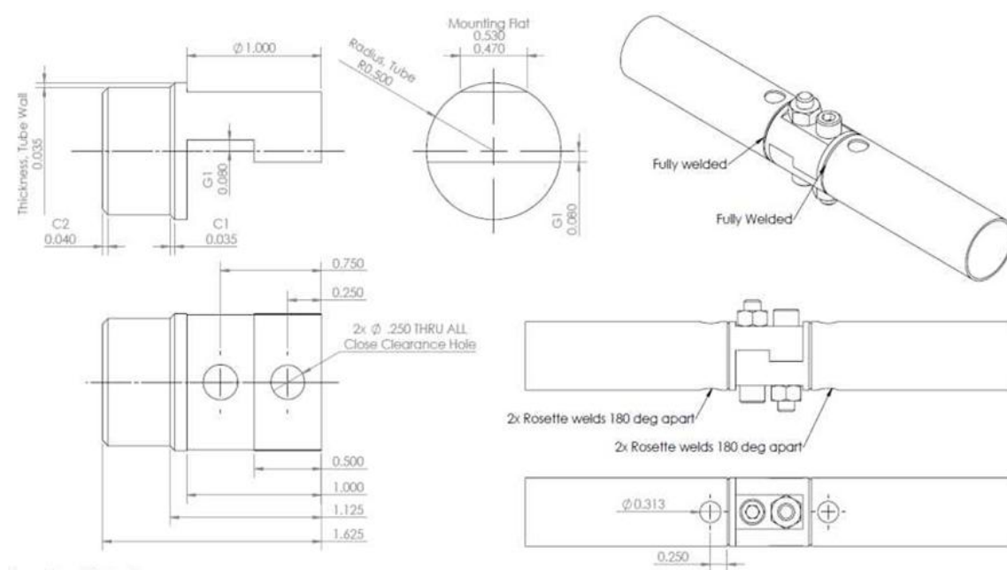
图B-37 防滚架 可拆卸构件接头
