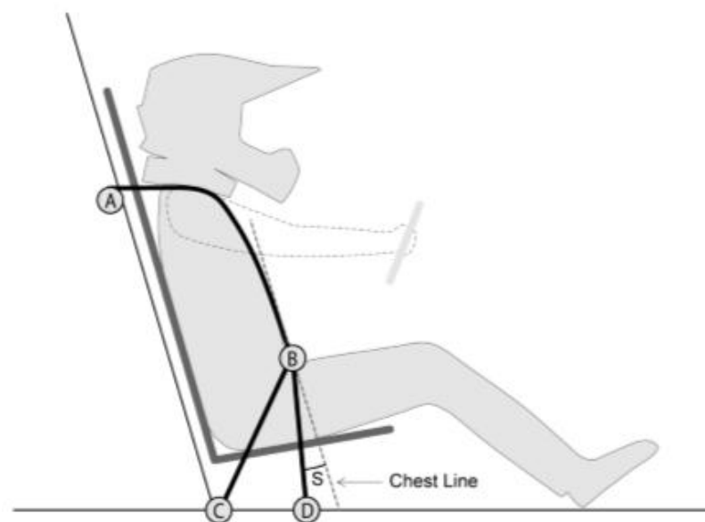
图B-48 车手安全带，反潜带角度
