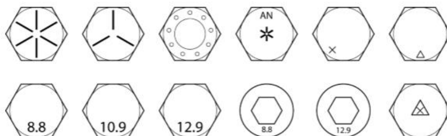
图B-69 紧固件，可接受的标记
