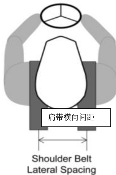
图B-43 车手背带、肩带横向位置
