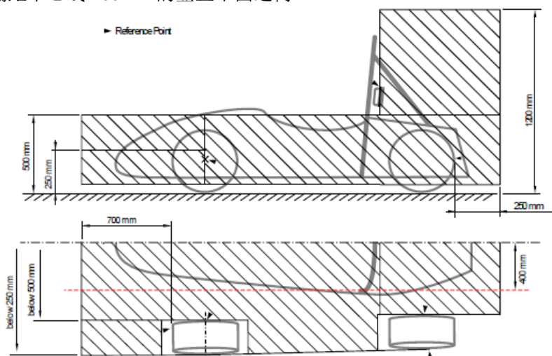
图2.26 空气动力学区域
