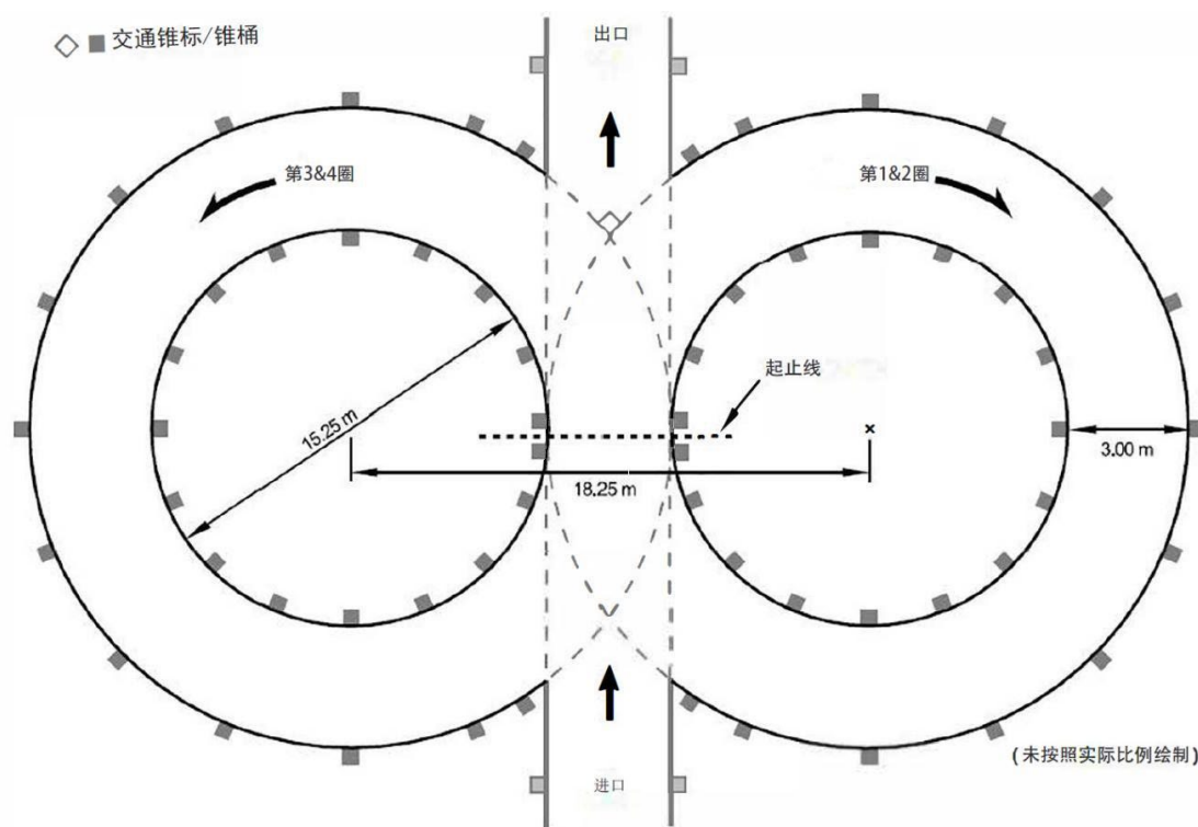
图8.3 八字赛道示意图
