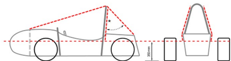
图 2.4 部件包络面示意图
