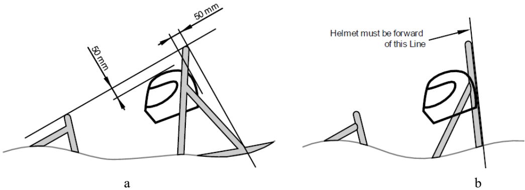
图 2.7 防滚架位置要求
