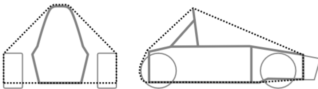
图 4.10 混合动力元件允许布置的区域
