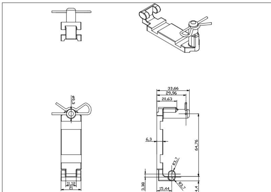
图 2.28 无线计时模块安装基座
