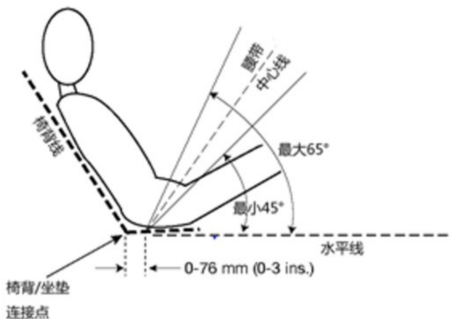
图 2.16 腰带的角度
