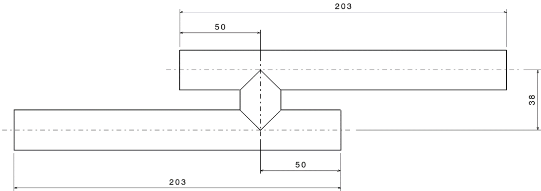
图 2.6 测试样管示意图
