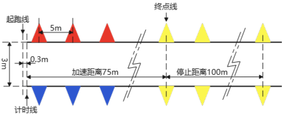
图 8.2 无人直线赛道示意图
