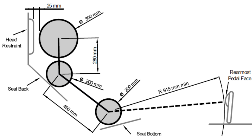
图 2.8 男性第 95 百分位模板位置
