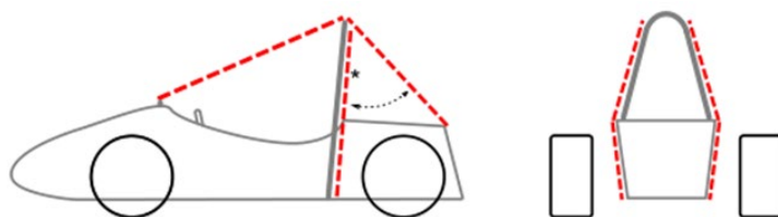
图 2.2 防滚架包络面示意图
