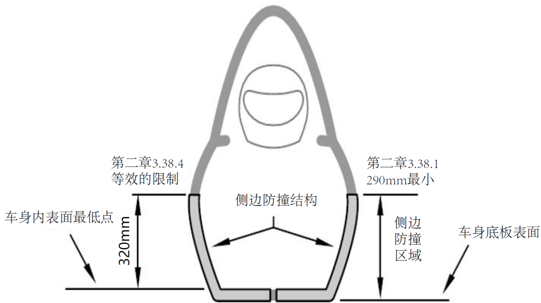
图 2.12 单体壳侧边防撞区域
