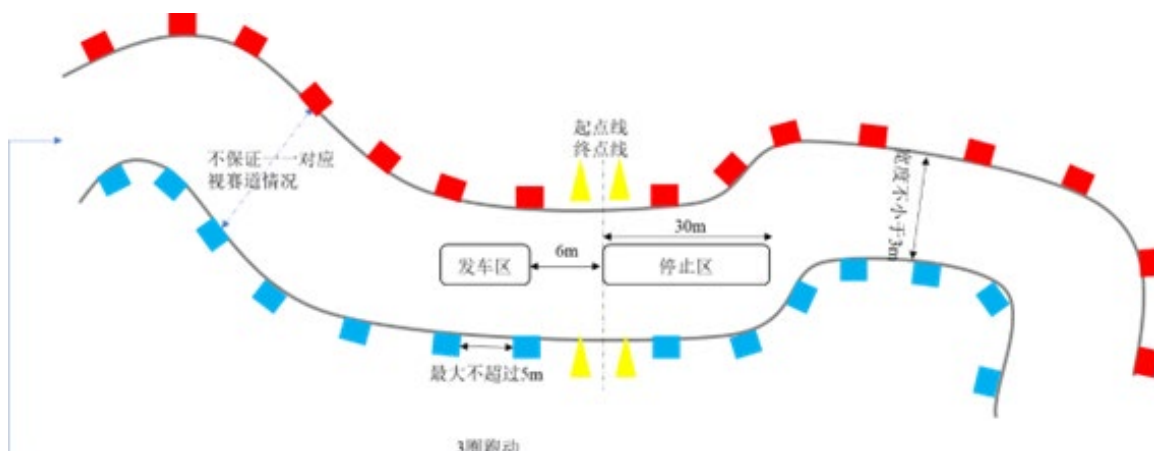
图 8.4: 高速循迹测试赛道示意图
