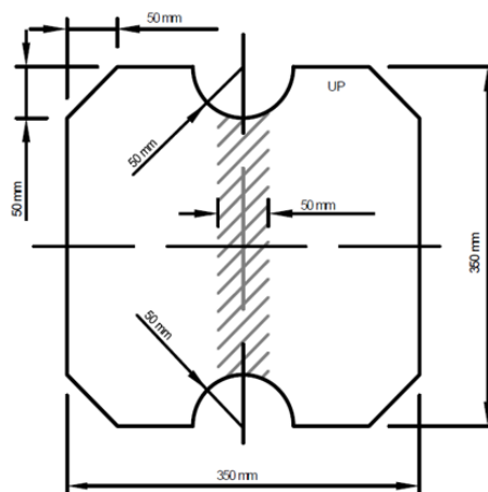
前舱检测板最大厚度：7mm
