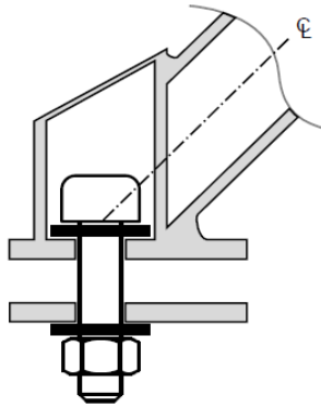
图 2.13 固定螺栓在管件中心线上
