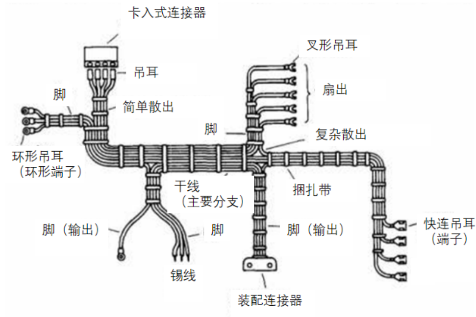
图 7.1 线束示意图
