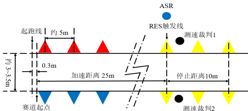
图2.23 EBS 测试赛道图
