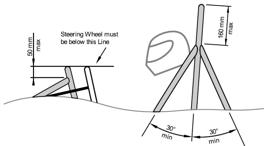
图 2.9 防滚架位置要求
