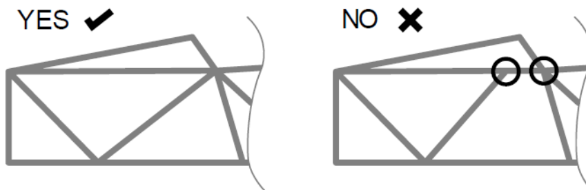
图 2.5 三角结构示例
