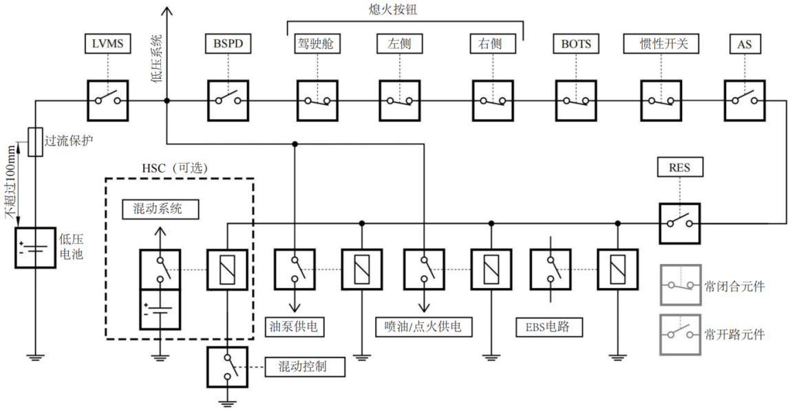
图 4.7 熄火电路示例原理图
