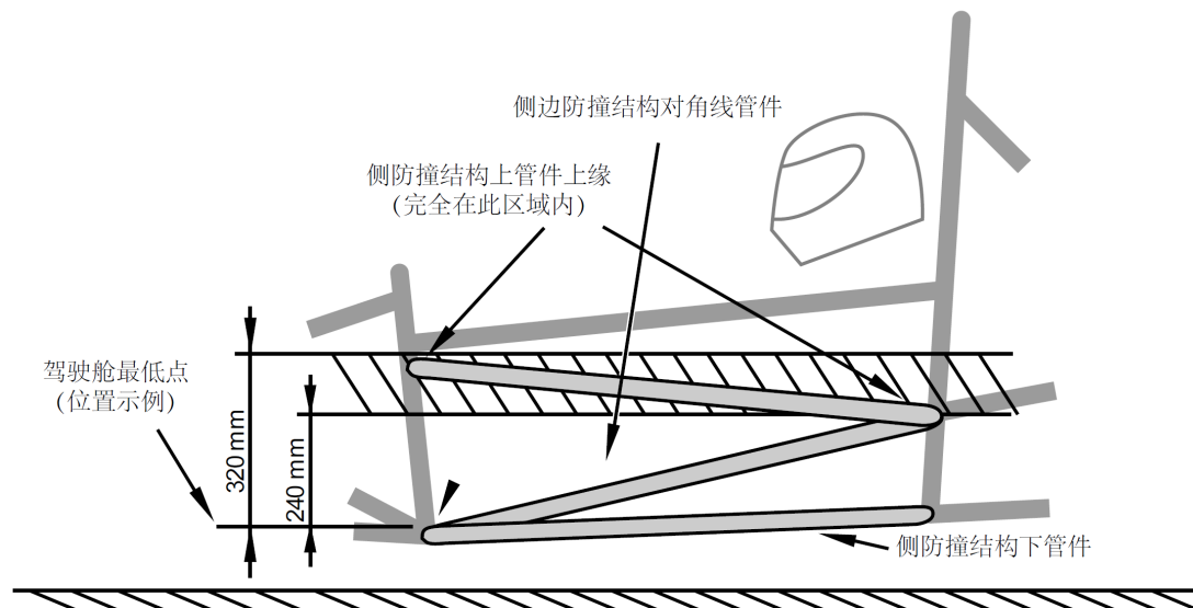
图 2.10 桁架式车架的侧边防撞结构
