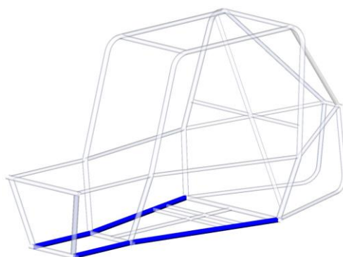
图B-27 LFS防滚架后支撑车架模式
