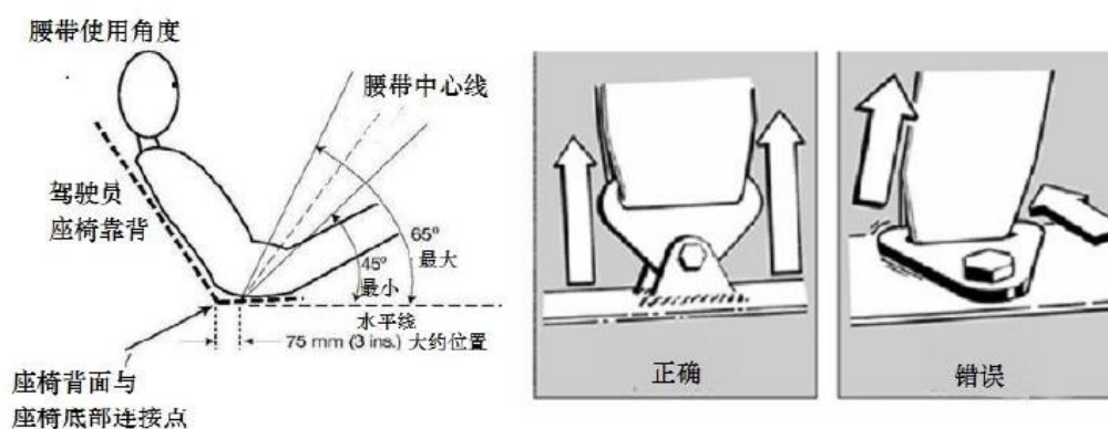
图B-47 车手安全带 搭扣方向
