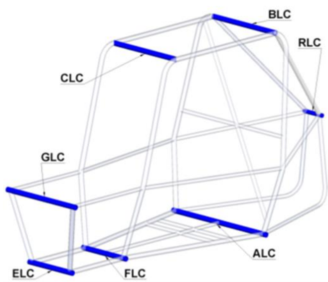
图 B-20 防滚架横向横梁 LC
