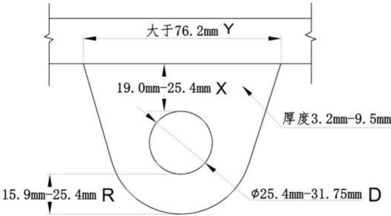
图B-67 后拖拽点尺寸图
