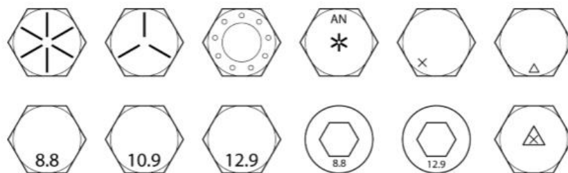
图B-69 紧固件，可接受的标记
