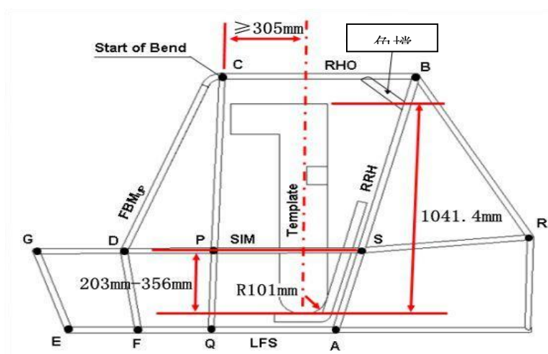
图B-24 防滚架 模板安装图
