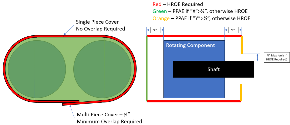
图B-60 动力传动系统CVT总成防护示例
