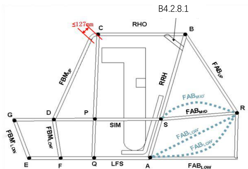
图B-32防滚架FAB
