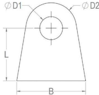
图B-70 吊耳几何形状
