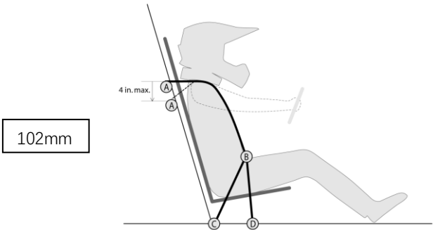
图B-42 安全带肩带垂直位置
