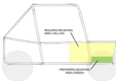
图B-75 应答器安装位置
