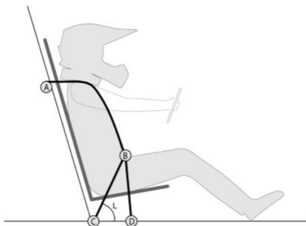
图B-46 车手安全腰带角度
