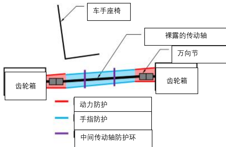
图B-61 中间传动轴防护
