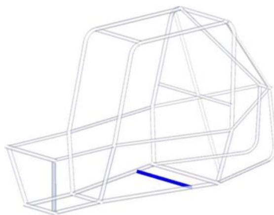
图B-29 防滚架USM示例
