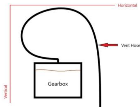
图B-62 空气收集系统通风管路布置（水平=从左到右）
