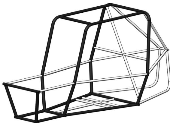
图B-17 防滚架主要构件(黑色填充)，后支撑车架
