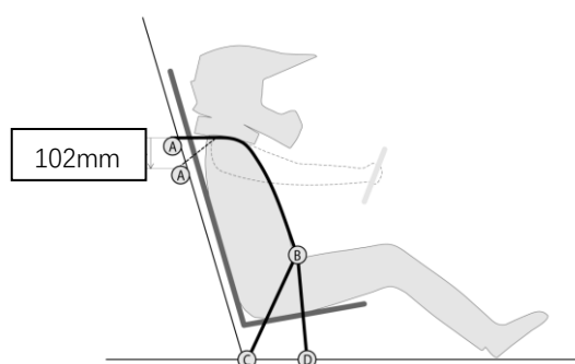
图B-46 安全带肩带垂直位置
